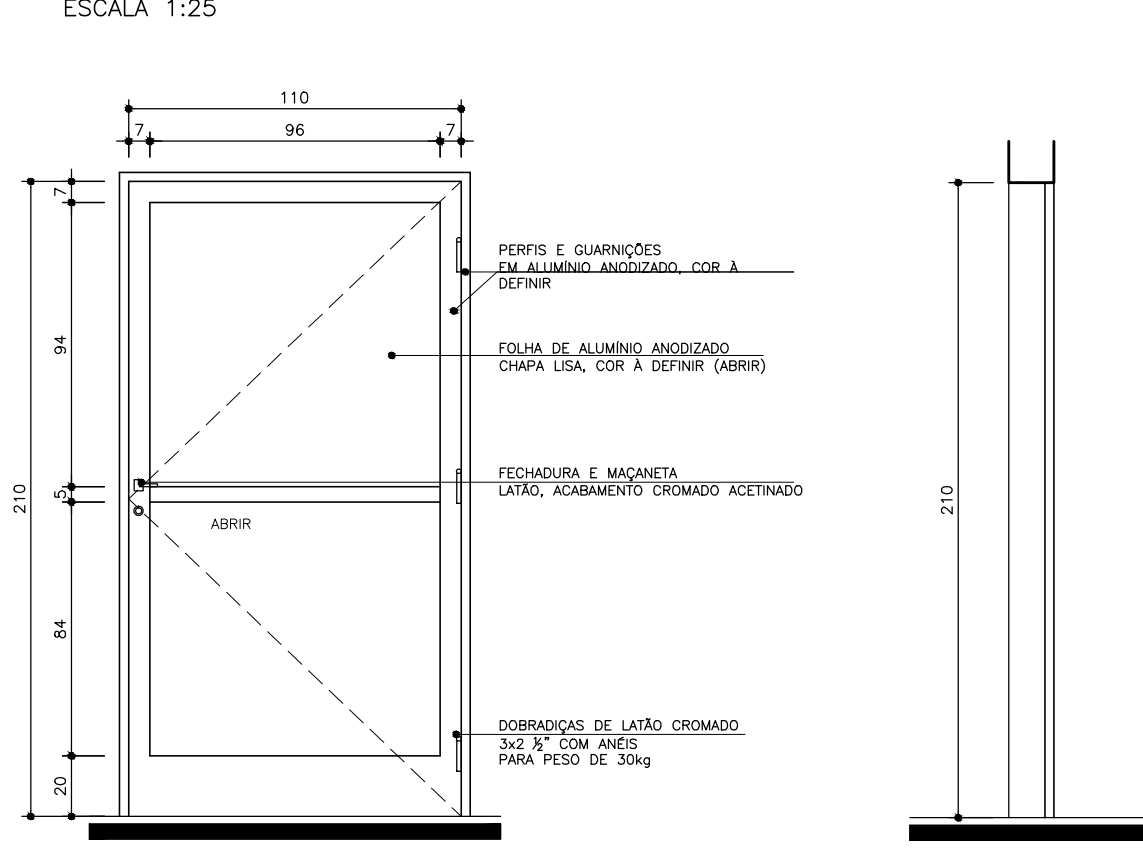
ELEVAÇÃO (PA/06) SEÇÃO (PA/06) ESCALA 1:25 ESCALA 1:25
