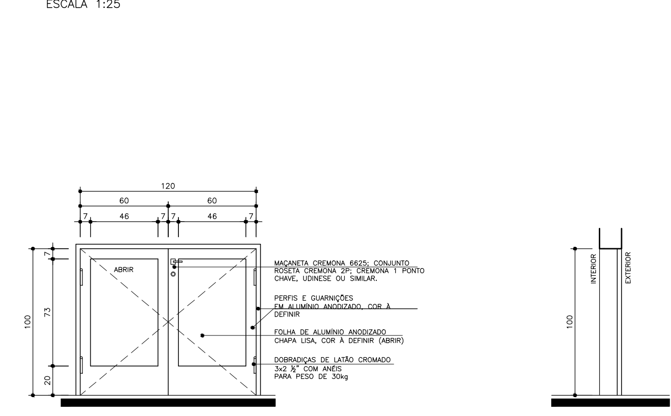
ELEVAÇÃO (PA/03) ESCALA 1:25 SEÇÃO (PA/03) ESCALA 1:25
