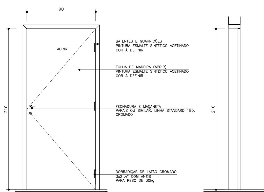
ELEVAÇÃO (PM/02) SEÇÃO (PM/02) ESCALA 1:25 ESCALA 1:25
