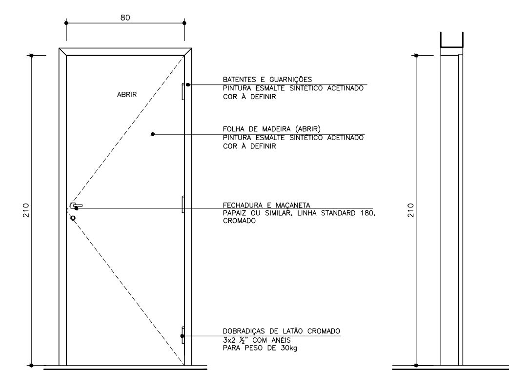
ELEVAÇÃO (PM/01) ESCALA 1:25 SEÇÃO (PM/01) ESCALA 1:25
