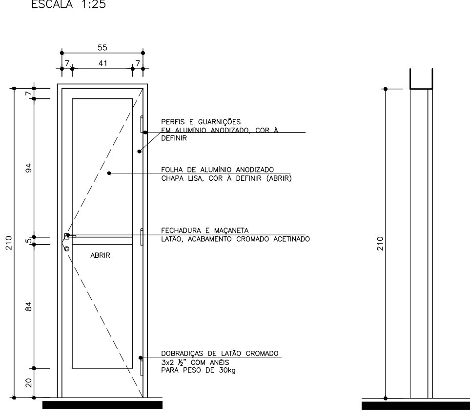
ELEVAÇÃO (PA/04) SEÇÃO (PA/04) ESCALA 1:25 ESCALA 1:25
