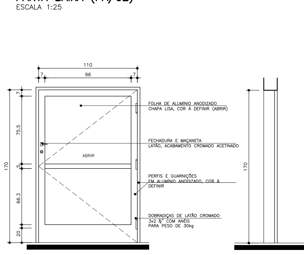
ELEVAÇÃO (PA/02) SEÇÃO (PA/02) ESCALA 1:25 ESCALA 1:25
