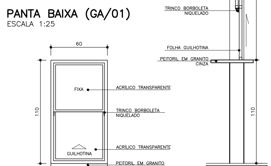
ELEVAÇÃO (GA/01) ESCALA 1:25
