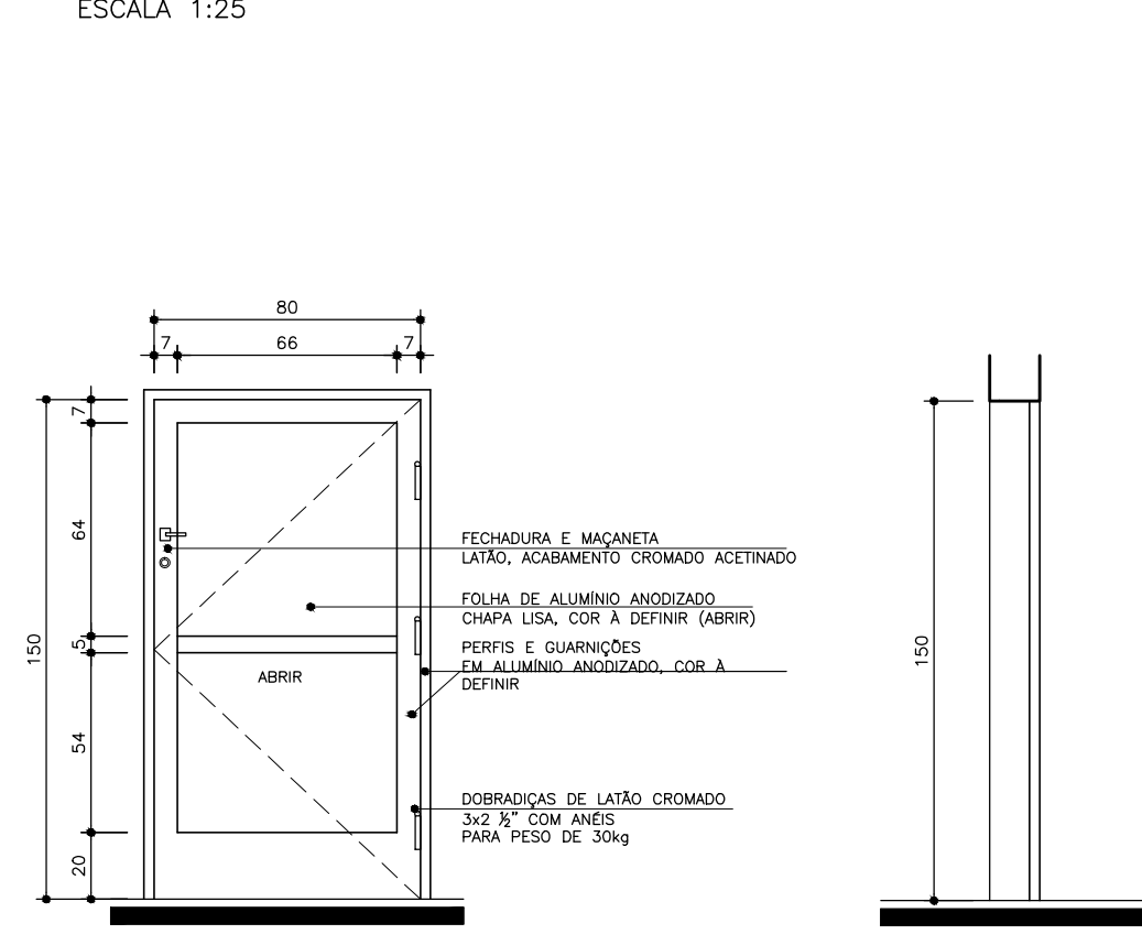
ELEVAÇÃO (PA/05) SEÇÃO (PA/05) ESCALA 1:25 ESCALA 1:25
