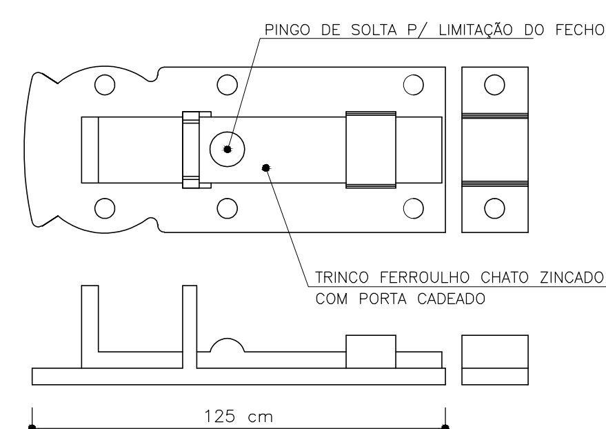
DET. TRINCO FERROHO SEM ESCALA
