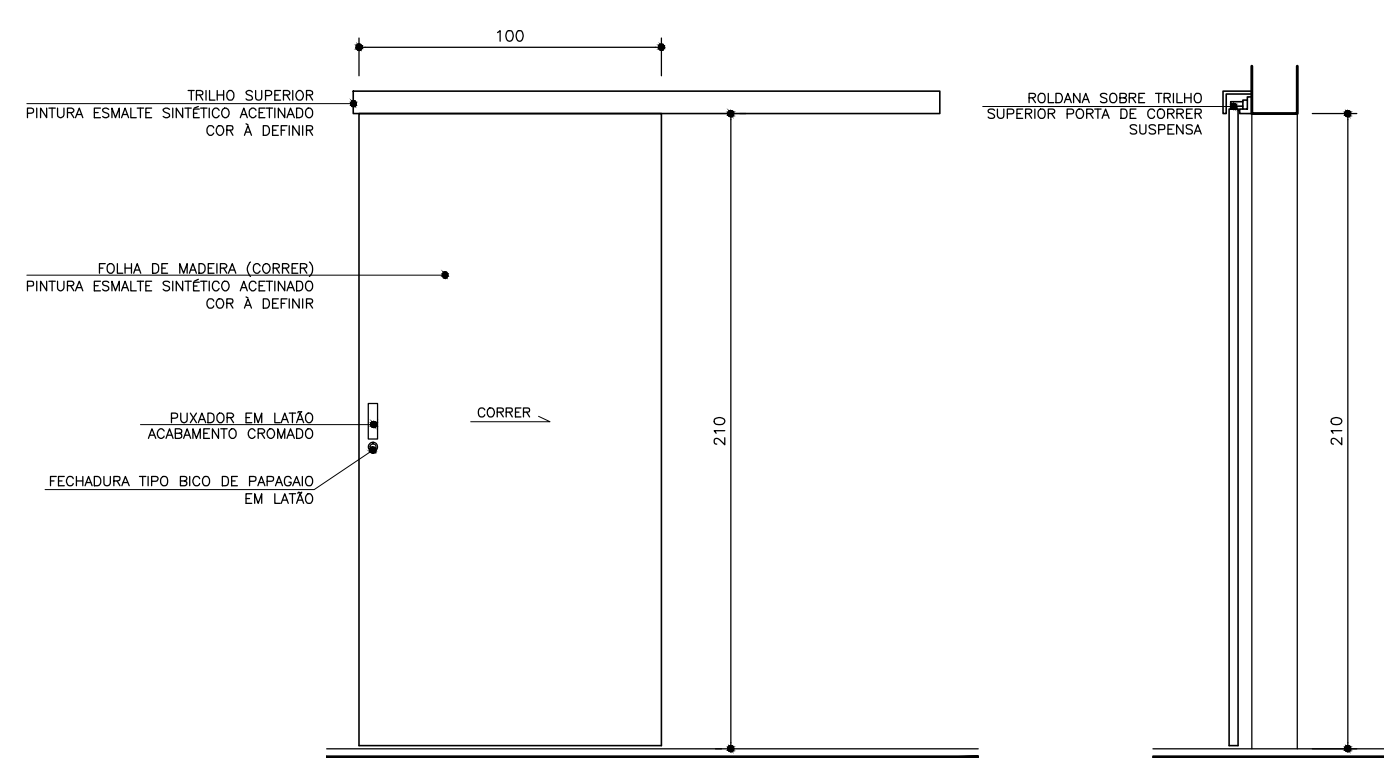
ELEVAÇÃO (PM/03) SEÇÃO (PM/03) ESCALA 1:25 ESCALA 1:25
