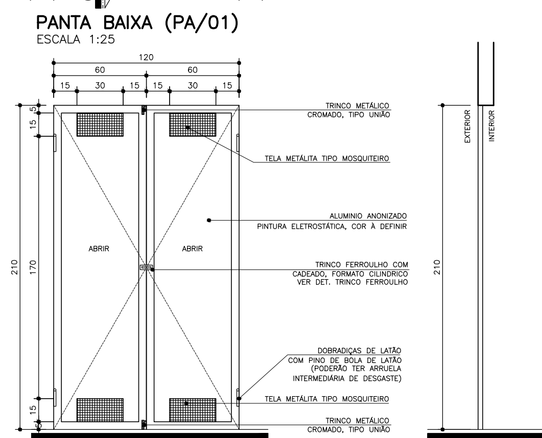
ELEVAÇÃO (PA/01) ESCALA 1:25
