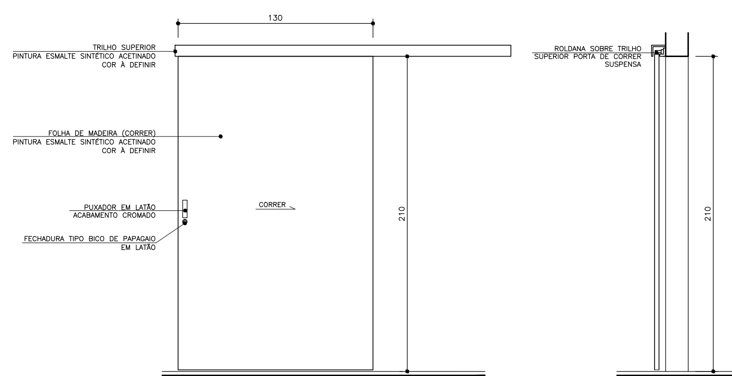
ELEVAÇÃO (PM/05) ESCALA 1:25 SEÇÃO (PM/05) ESCALA 1:25
