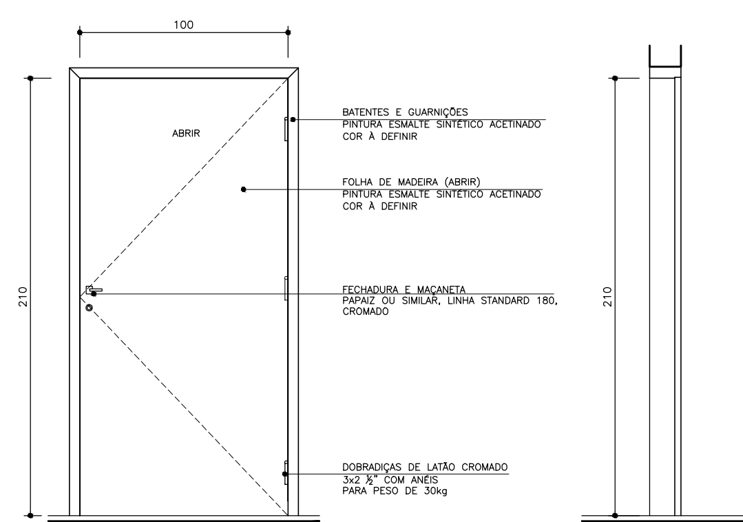
ELEVAÇÃO (PM/04) SEÇÃO (PM/04) ESCALA 1:25 ESCALA 1:25
