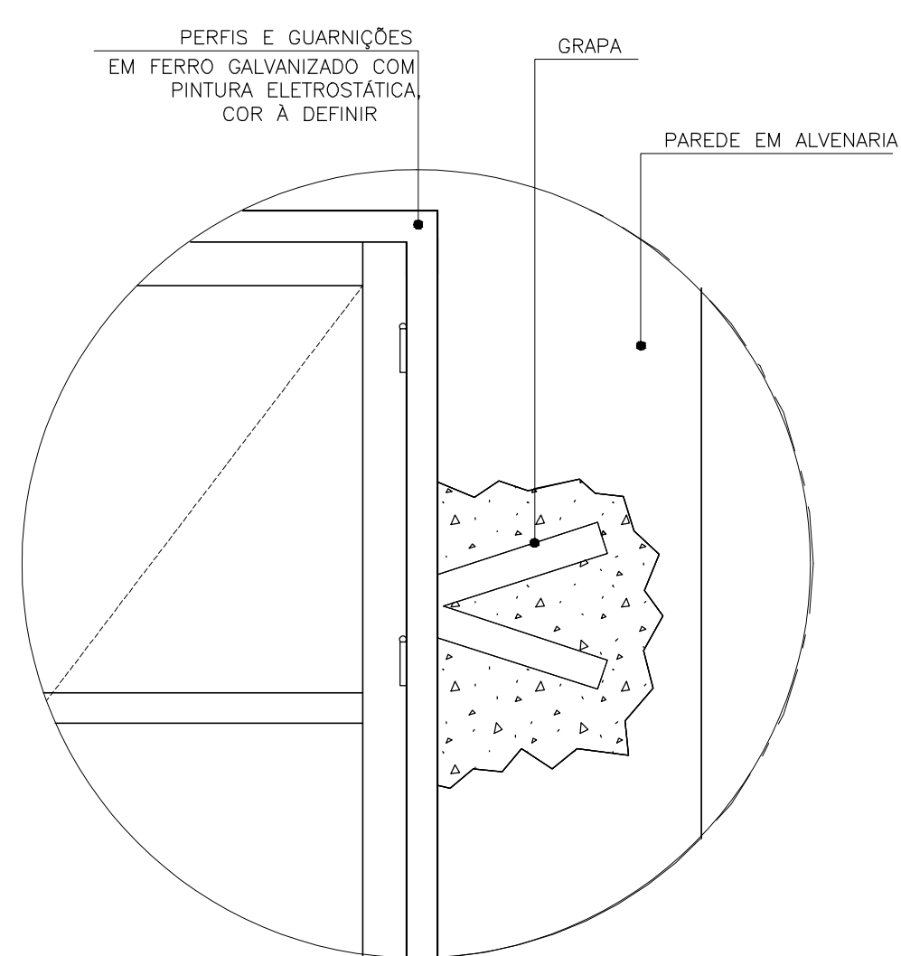
ELEVAÇÃO (PA/01) ESCALA 1:25
