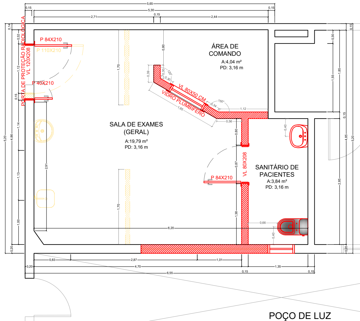
PLANTA DE DEMOLIR E CONSTRUIR ESC: 1/50
