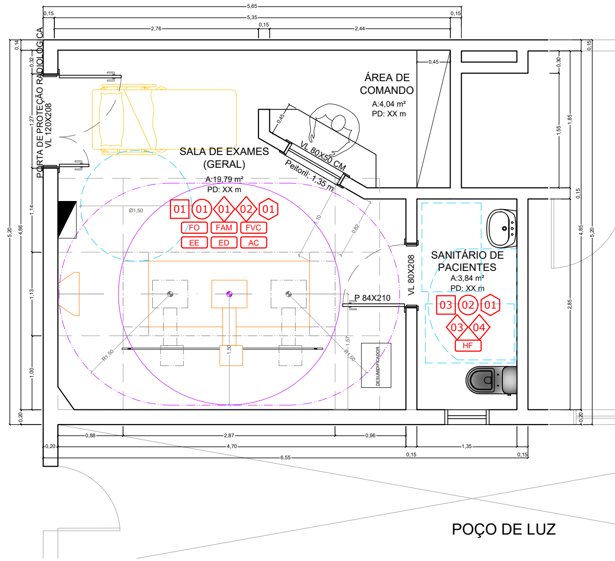
PLANTA BAIXA 1º PAVIMENTO ESC: 1/50
