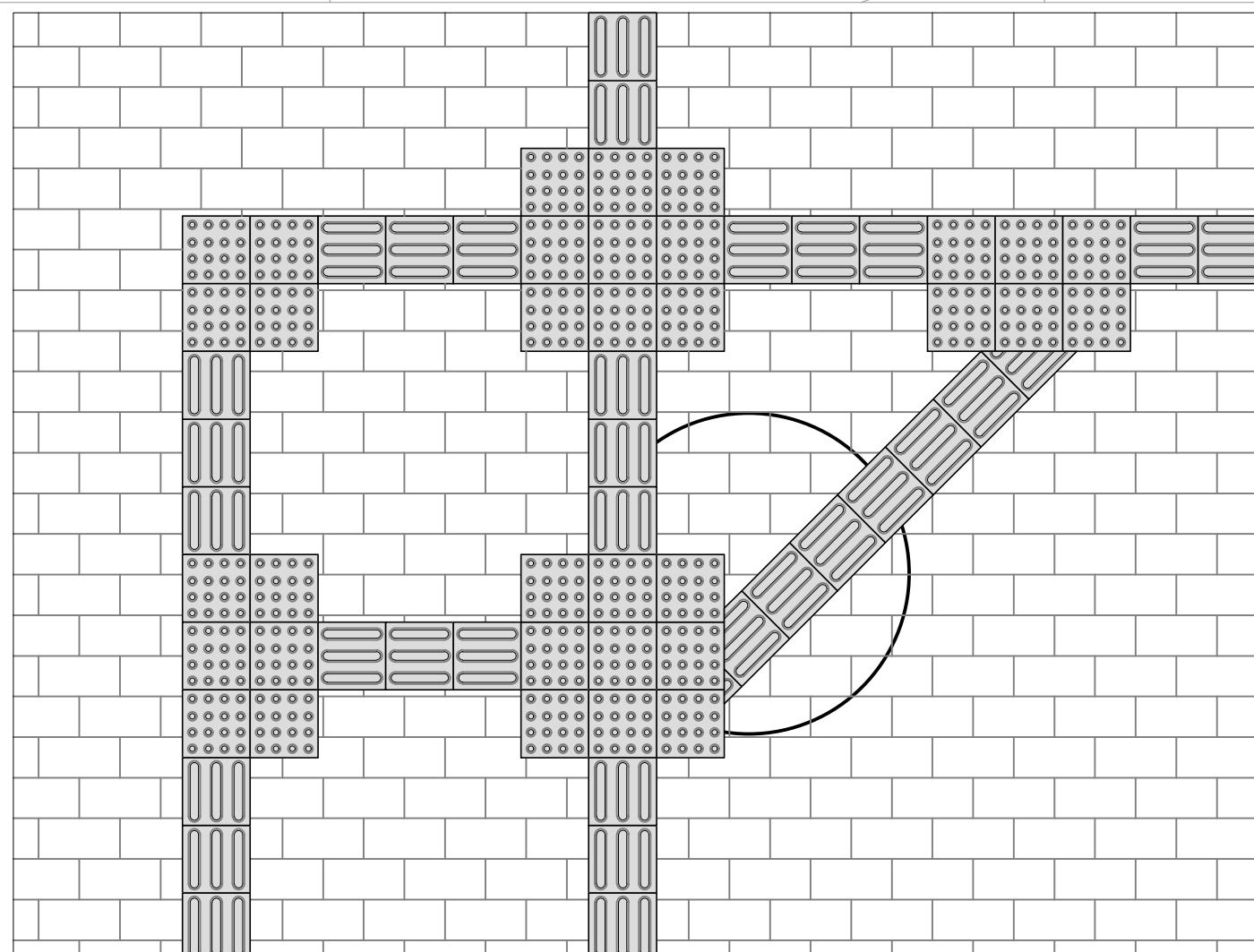
Composição de sinalização tátil de alerta e direcional - Exemplo
