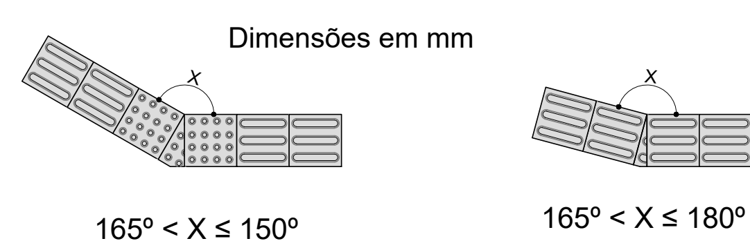
Composição de sinalização tátil de alerta e direcional Exemplo de mudanças de direção
