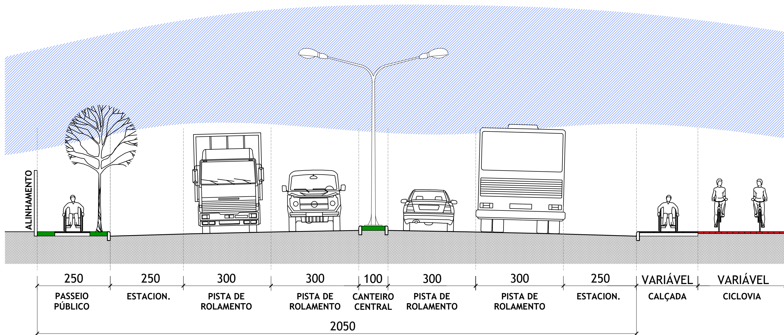
PERFIL VIÁRIO (URBANÍSTICO) - 1/75
