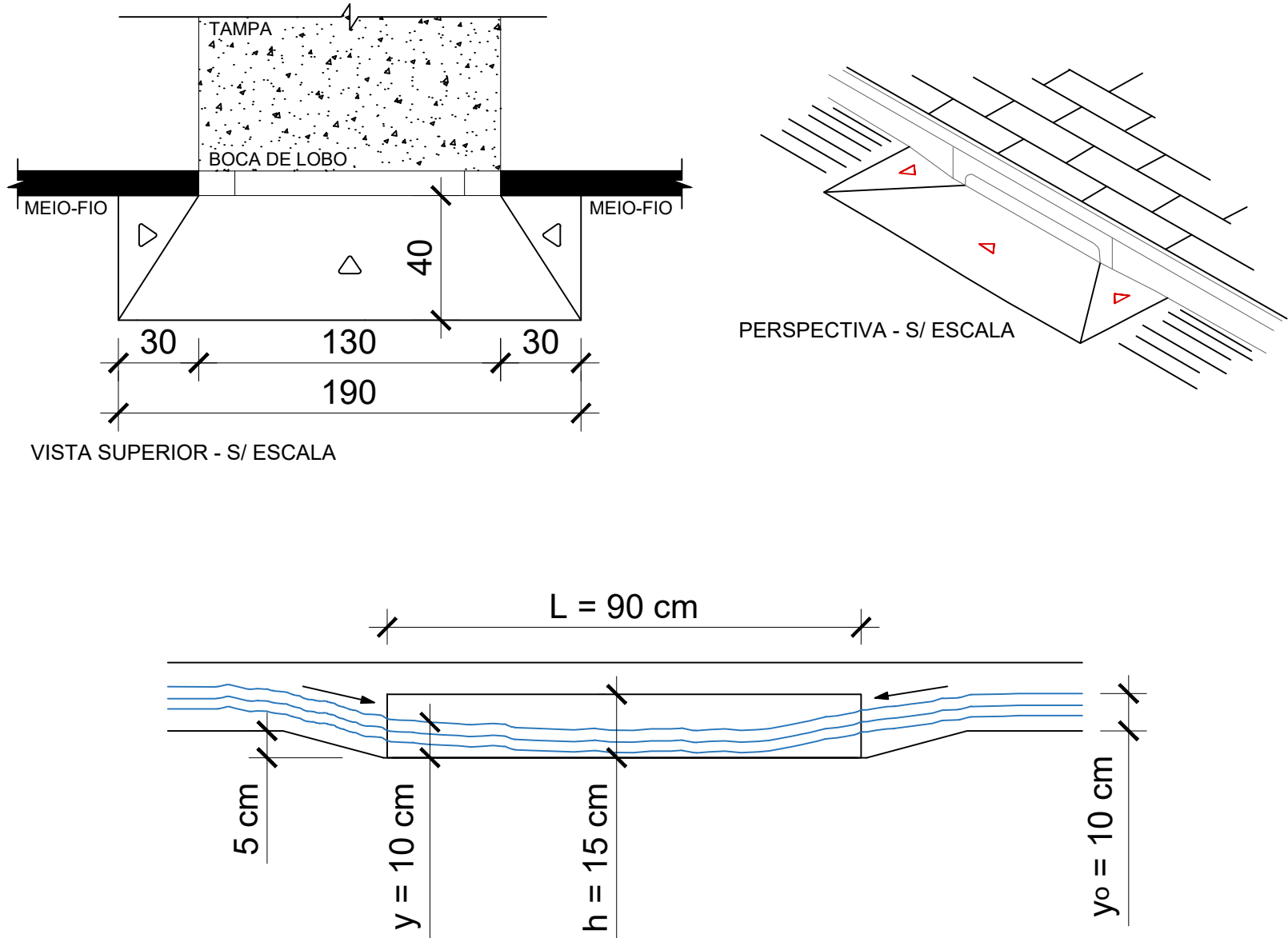
DETALHAMENTO DE REBAIXO DO PAVIMENTO NAS BOCAS DE LOBO - SEM ESCALA -
