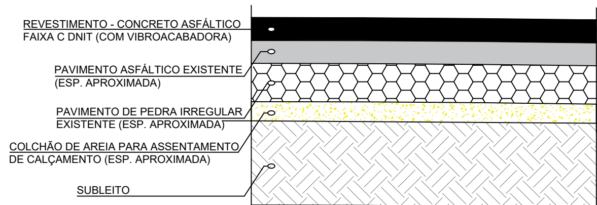
DETALHAMENTO CAMADAS - SEM ESCALA -
