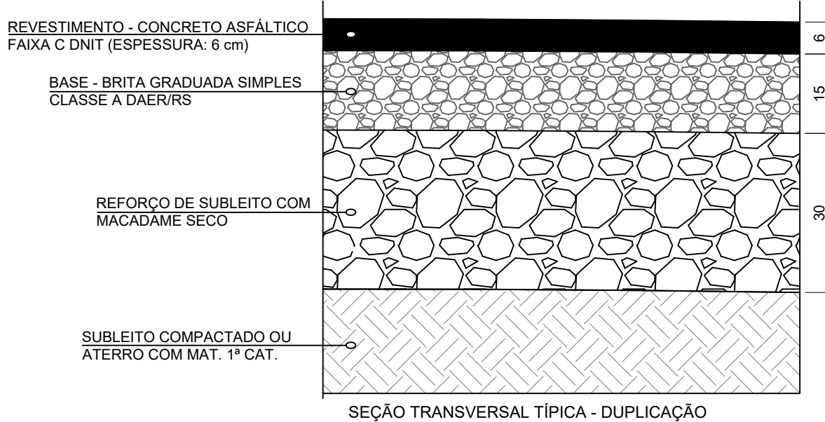
DETALHAMENTO CAMADAS - SEM ESCALA -
