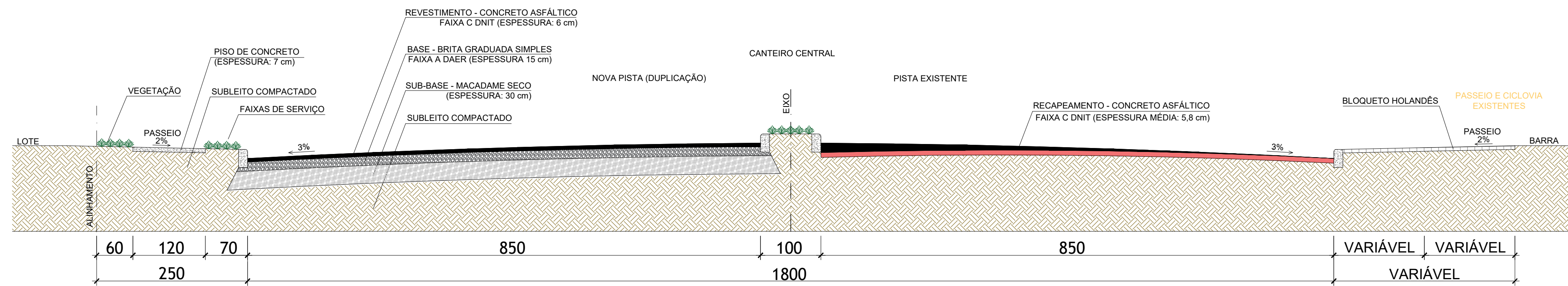
SEÇÃO TIPO - 1/50
