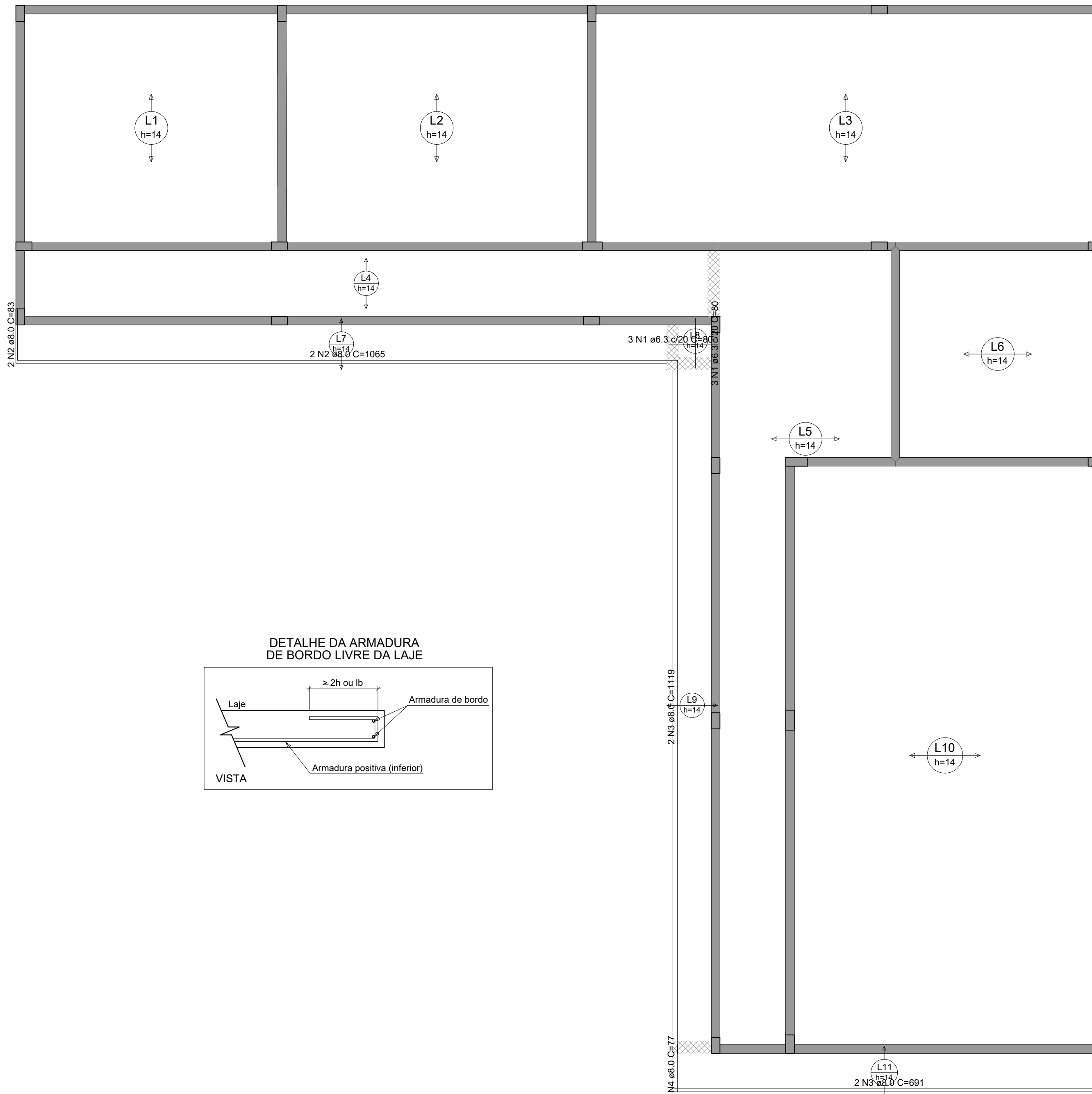
ARMAÇÃO POSITIVA DAS LAJES DO PAVIMENTO TETO (EIXO X / EIXO Y)
