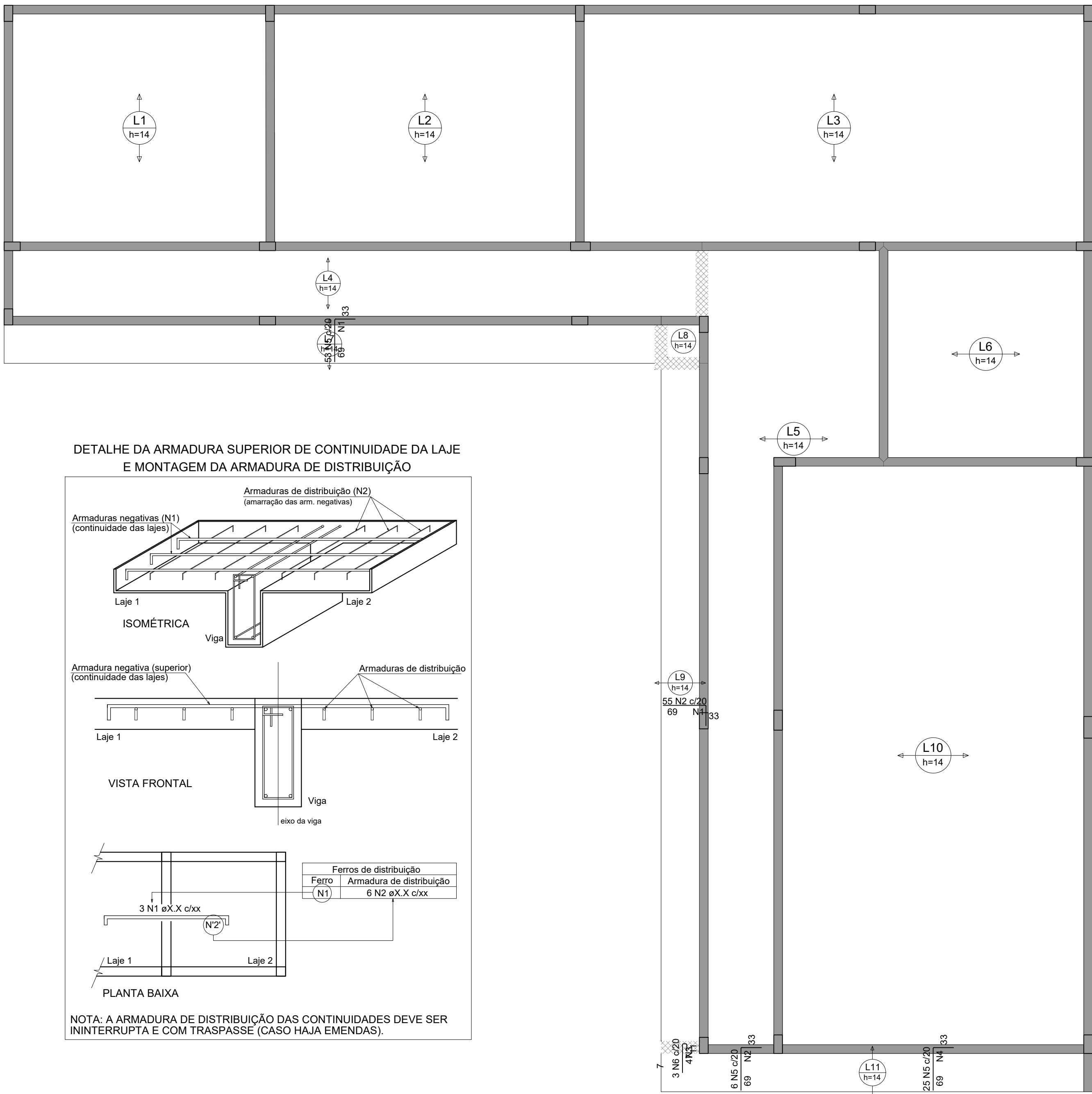
ARMAÇÃO NEGATIVA DAS LAJES DO PAVIMENTO TETO (EIXO X / EIXO Y)
