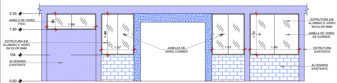
CORTE A-A
