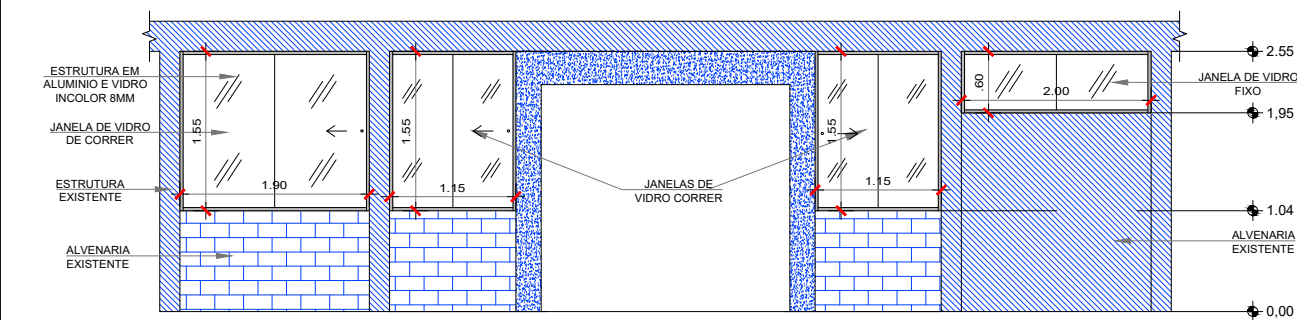
CORTE B-B
