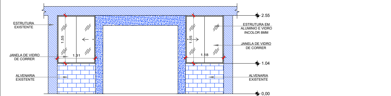
CORTE C-C
