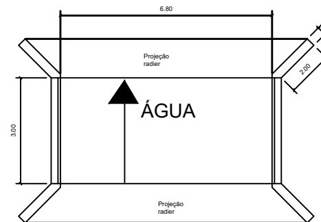
Planta Baixa
