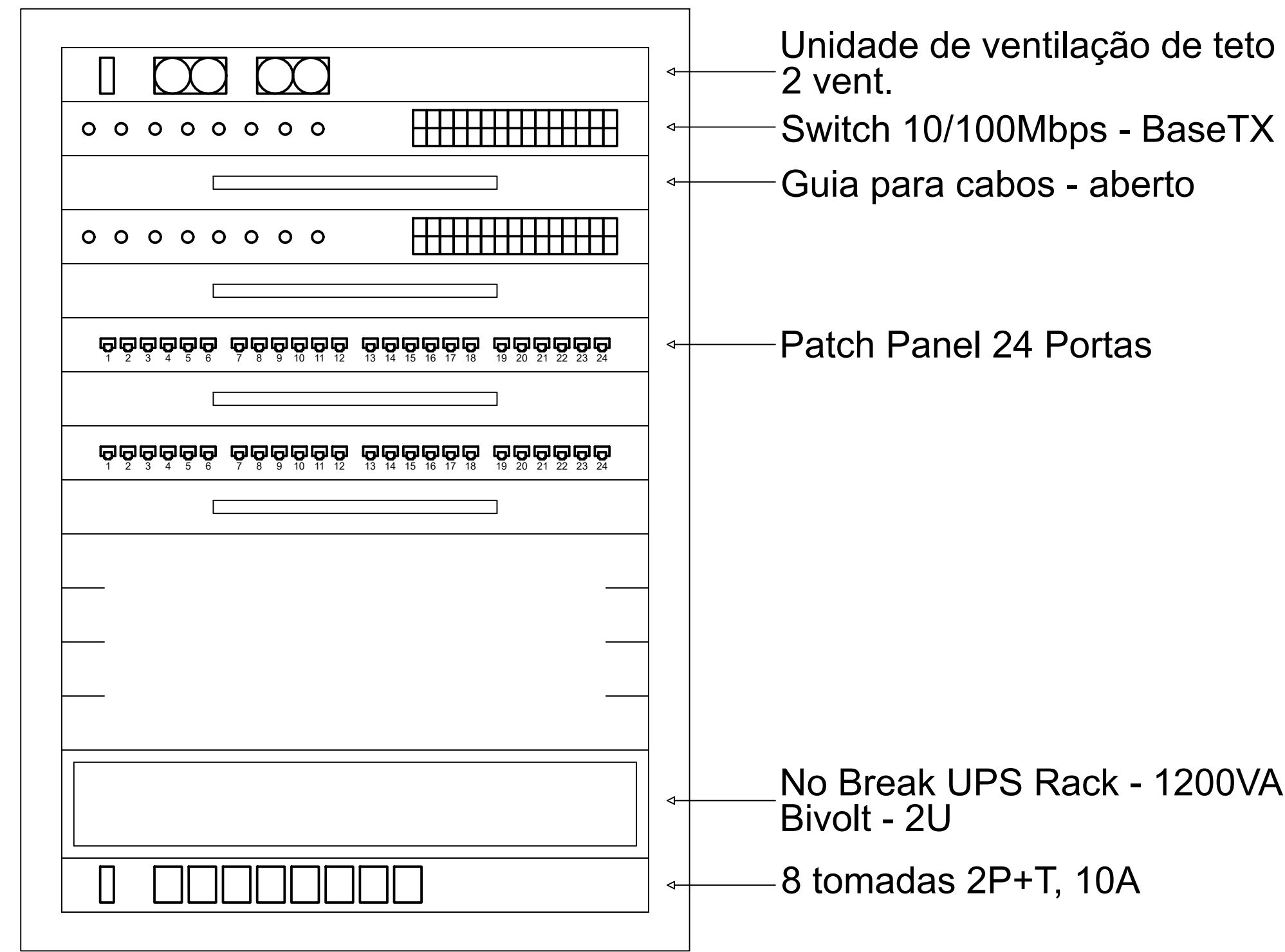
DETALHE 01 Plano de face do Rack
