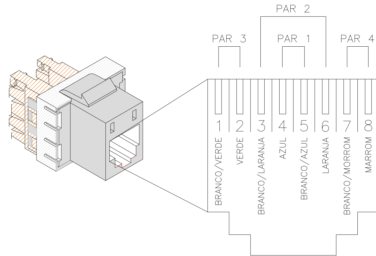
DETALHE 02 Ligação Conector do RJ45 Padrão
