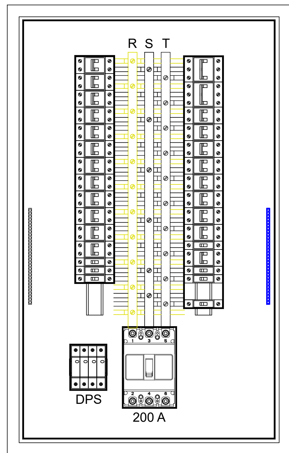
DETALHE 03 PLANO DE FACE QGBT
