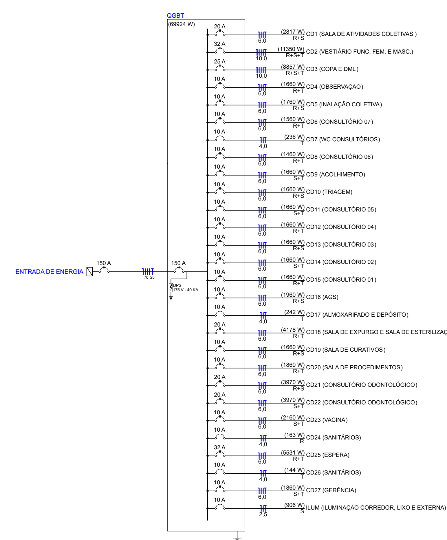
DETALHE 02 DIAGRAMA UNIFILAR
