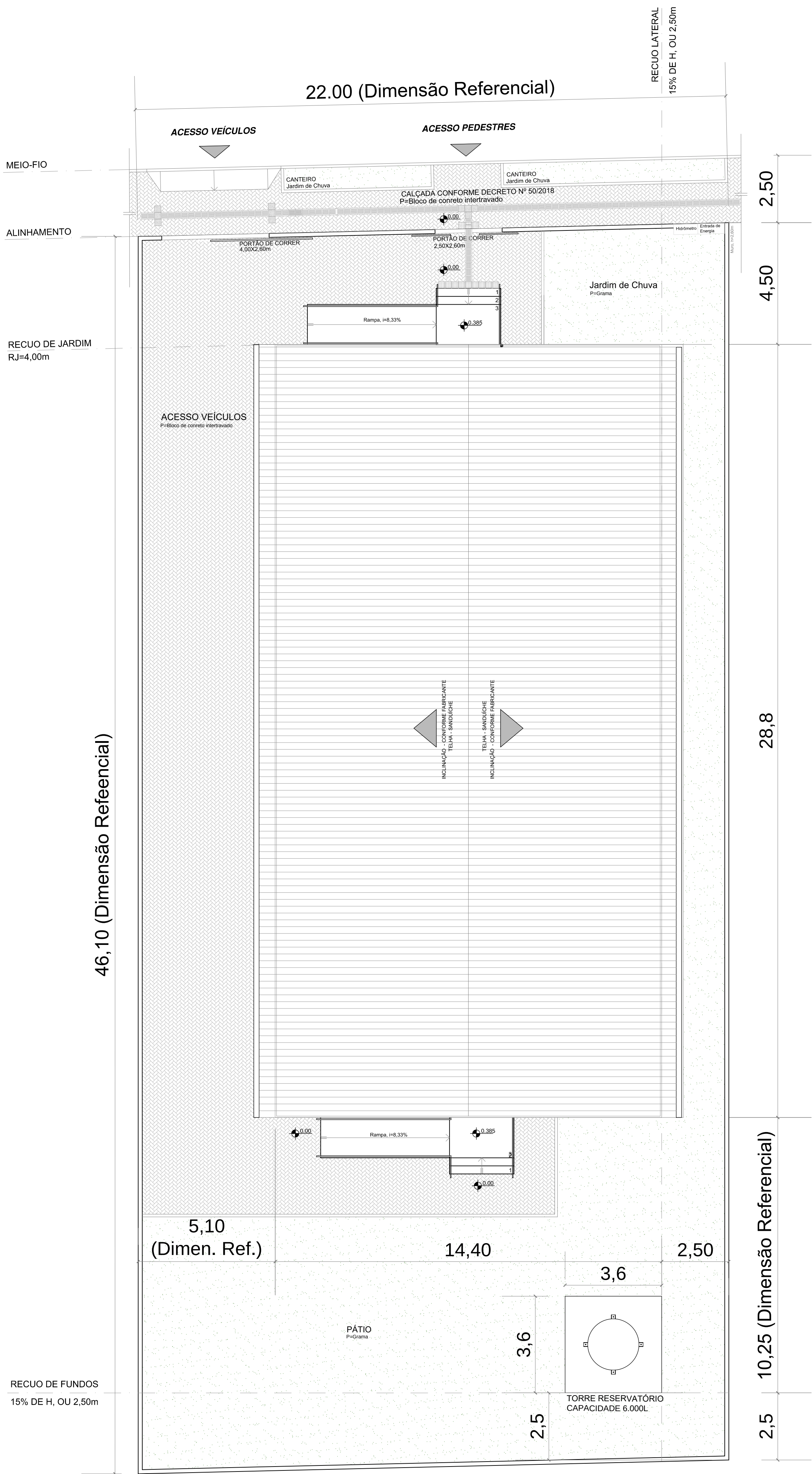
PLANTA DE IMPLANTAÇÃO ESC.1/100
