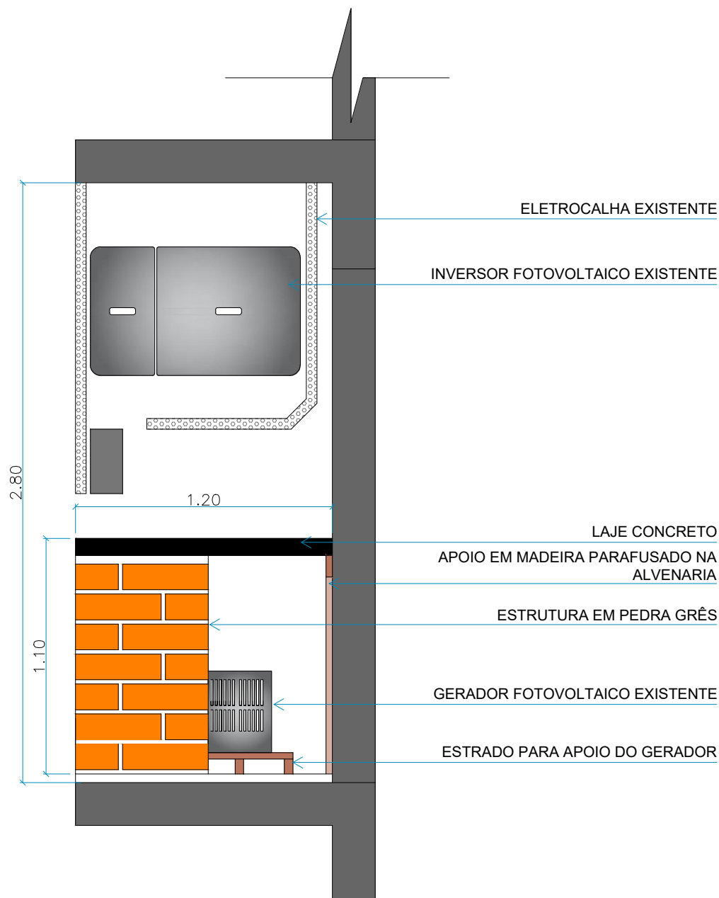
VISTA FRONTAL SITUAÇÃO ATUAL
