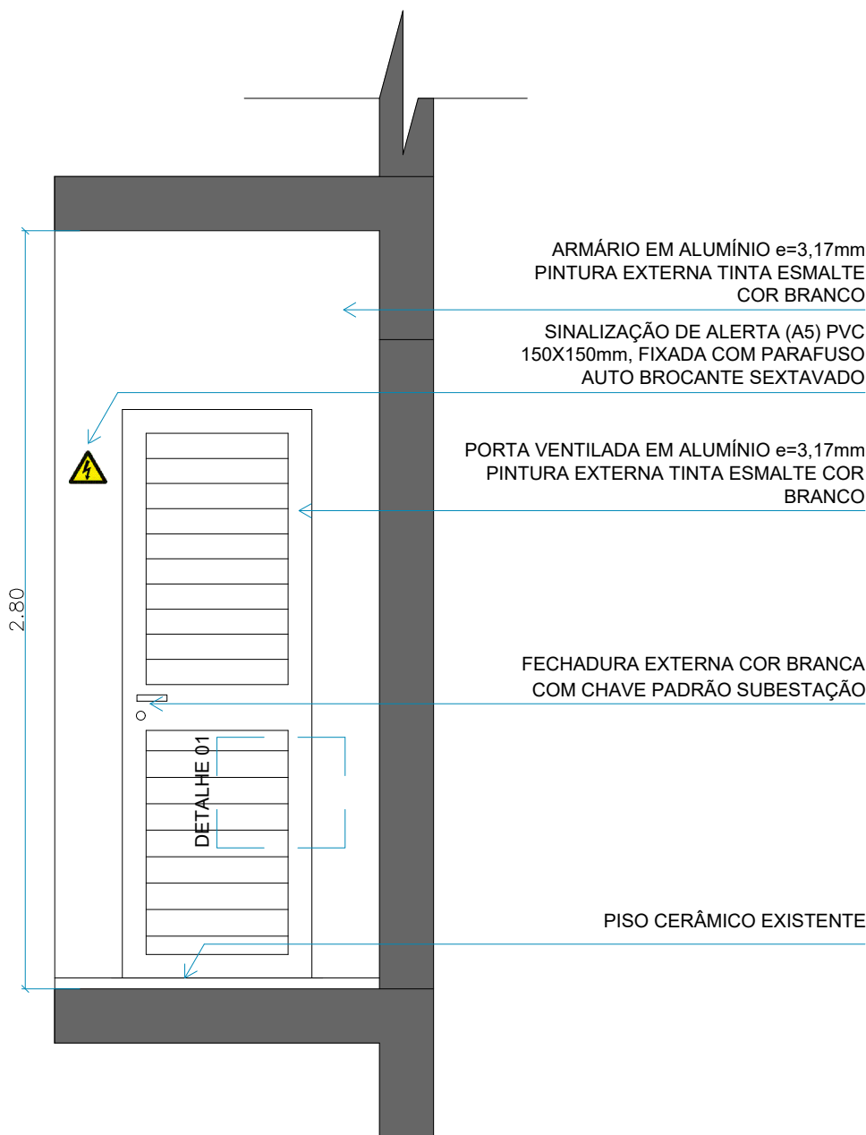
VISTA FRONTAL SITUAÇÃO PROPOSTA
