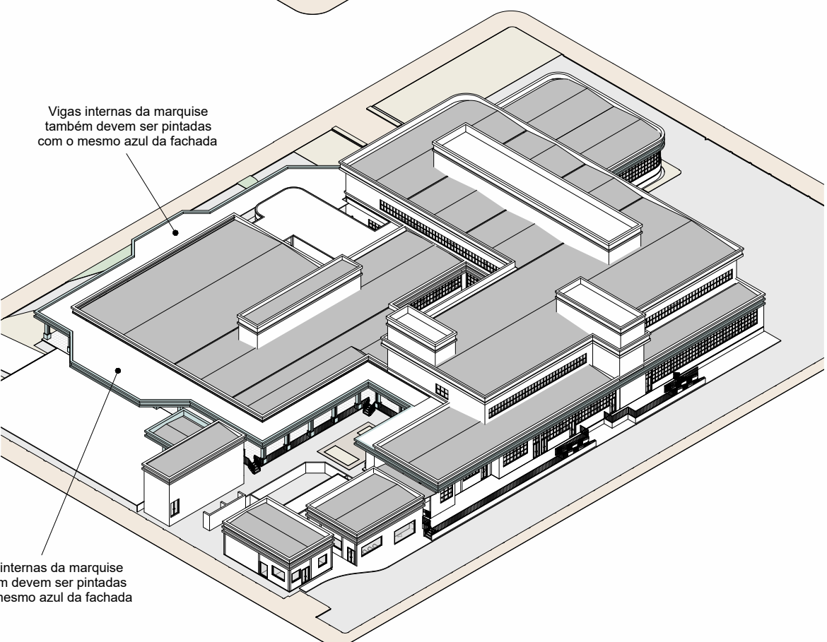
5 ISOMÉTRICAS 1:125
