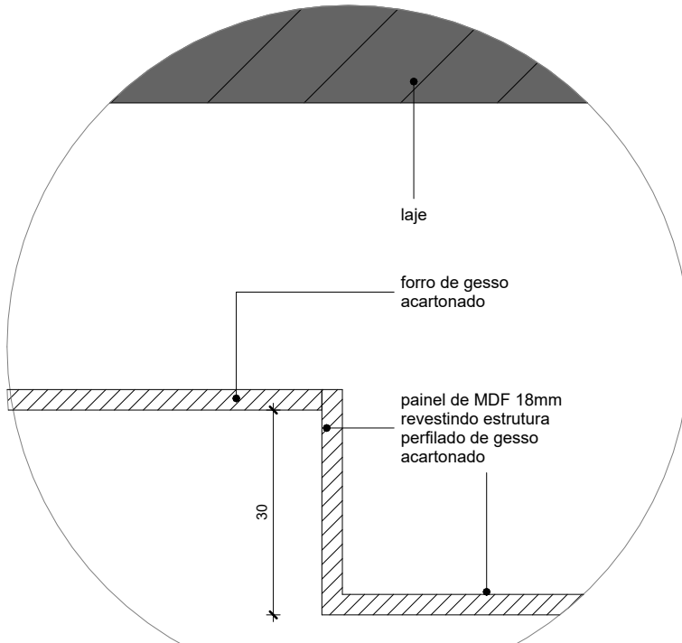
A DET-A - REBAIXO NO GESSO
