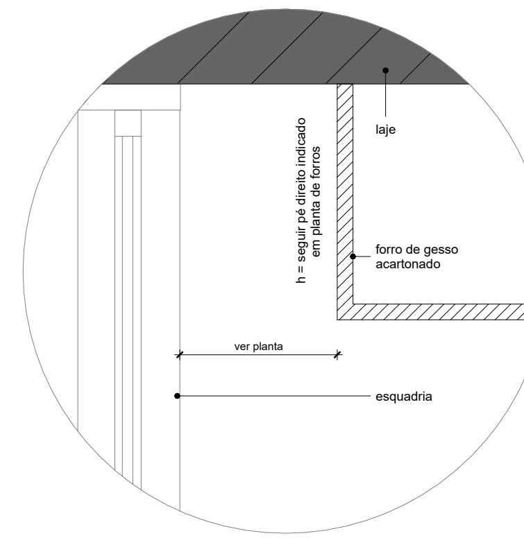
B DET-B - CORTINEIRO
