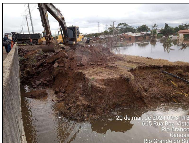
Figura 12: fechamento provisório dique Rio Branco
