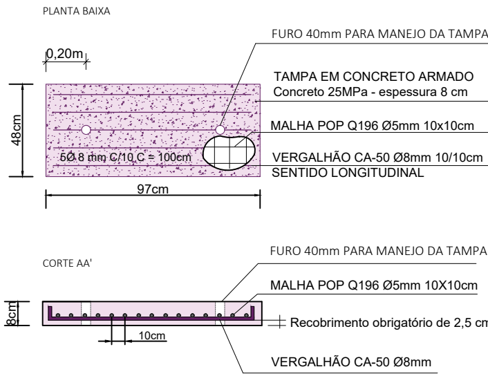
SEM ESCALA OBS.: Movimentar somente 14 dias após a concretagem. Mentir o concreto umedecido nos primeiros 7 dias.
