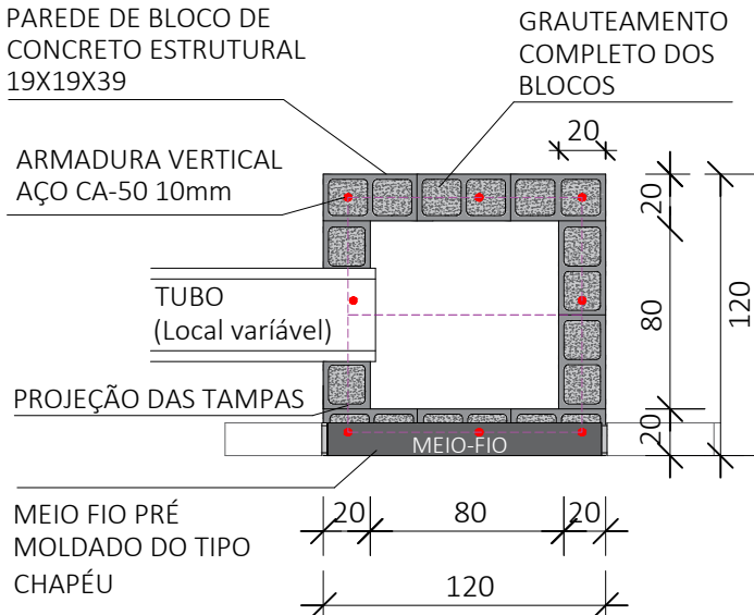
PLANTA BAIXA - Caixa BLS (0,80 x 0,80m) Sem escala Unidade: cm
