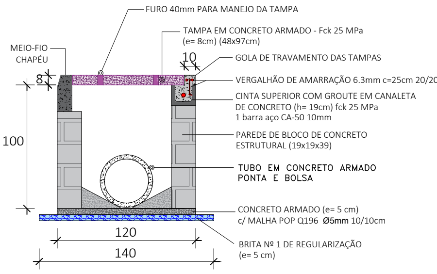
CORTE - Caixa BLS (1,00 x 1,00) Sem escala Unidade: cm
