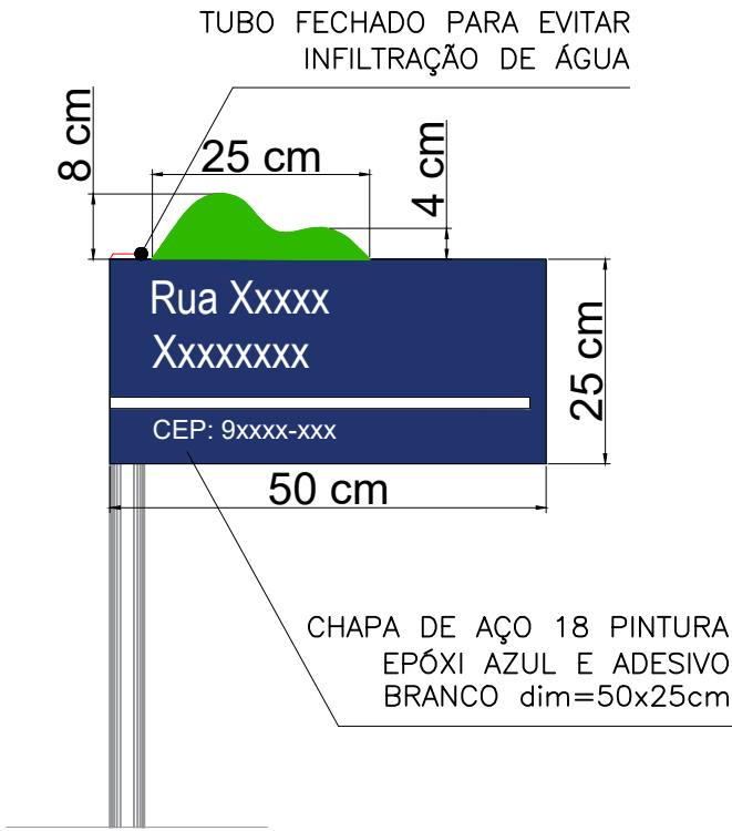
DETALHE PLACAS DE IDENTIFICAÇÃO DAS RUAS
