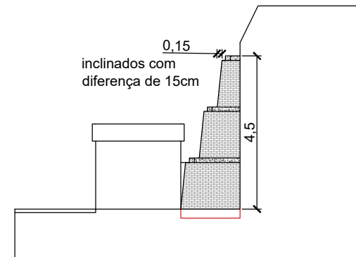
Corte
