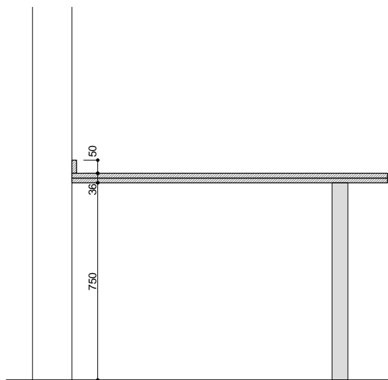
CORTE LONGITUDINAL
