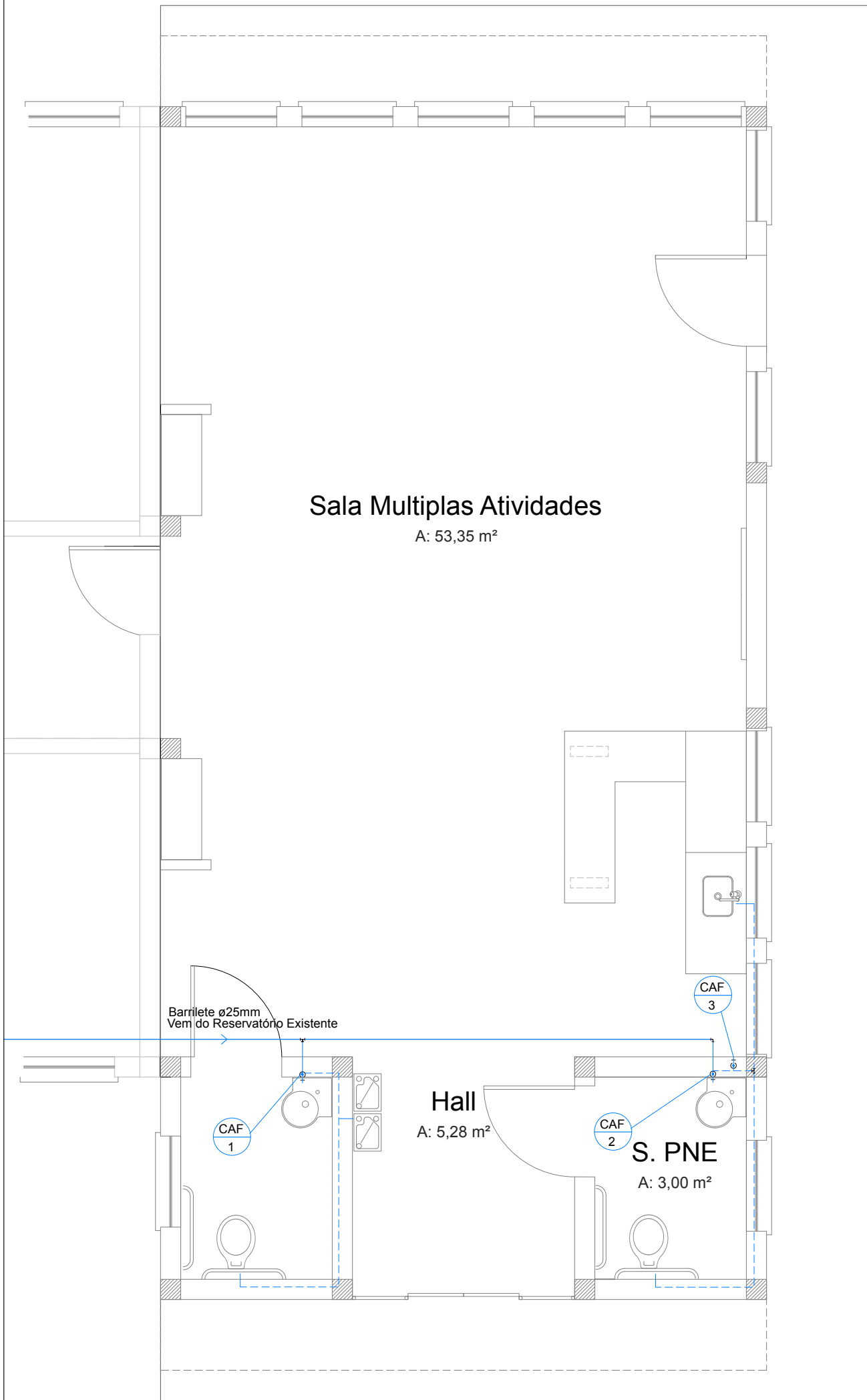
PLANTA BAIXA HIDRÁULICO ESCALA: 1/50
