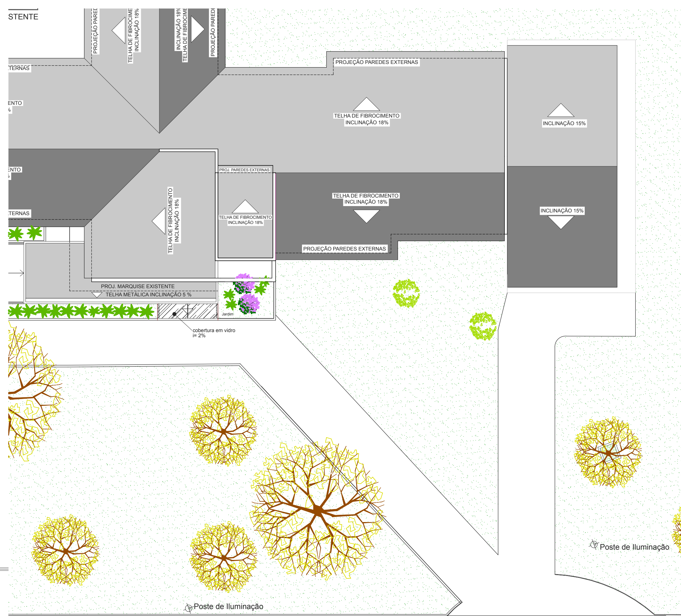
IMPLANTAÇÃO COM PLANTA DE COBERTURA ESCALA 1/125
