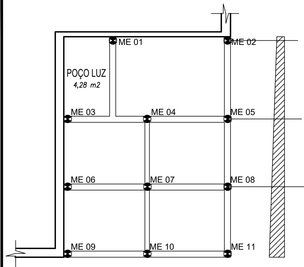
PLANTA BAIXA MICRO ESTACA/ BALDRAME
