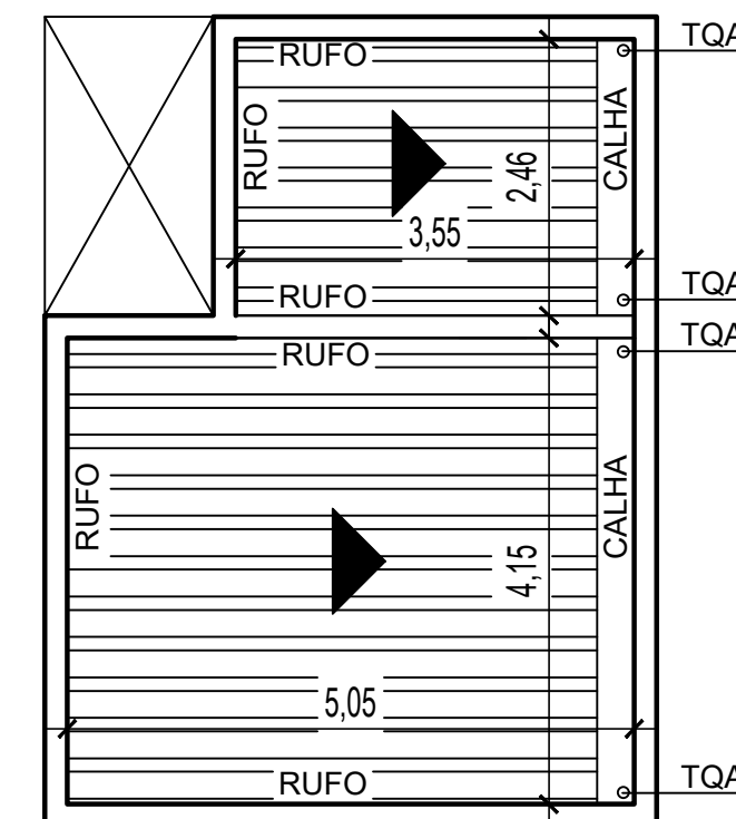
PLANTA BAIXA COBERTURA AMPLIAÇÃO
