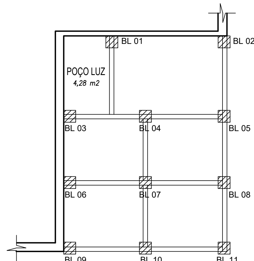
PLANTA BAIXA BLOCOS DE FUNDAÇÃO
