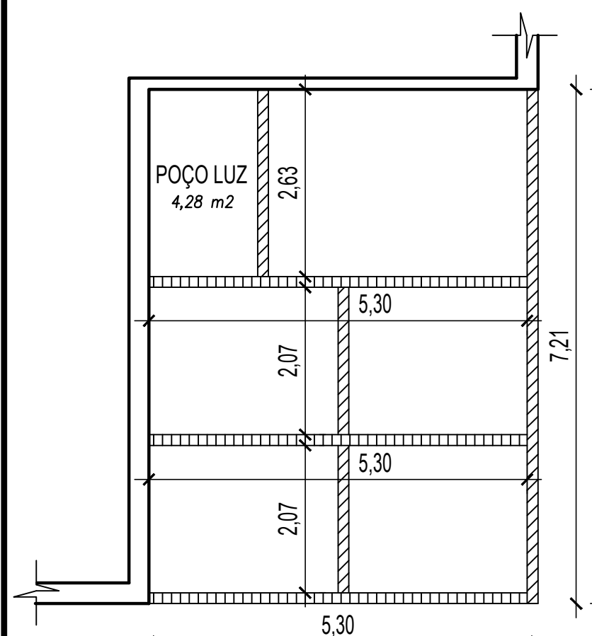
PLANTA BAIXA BALDRAME
