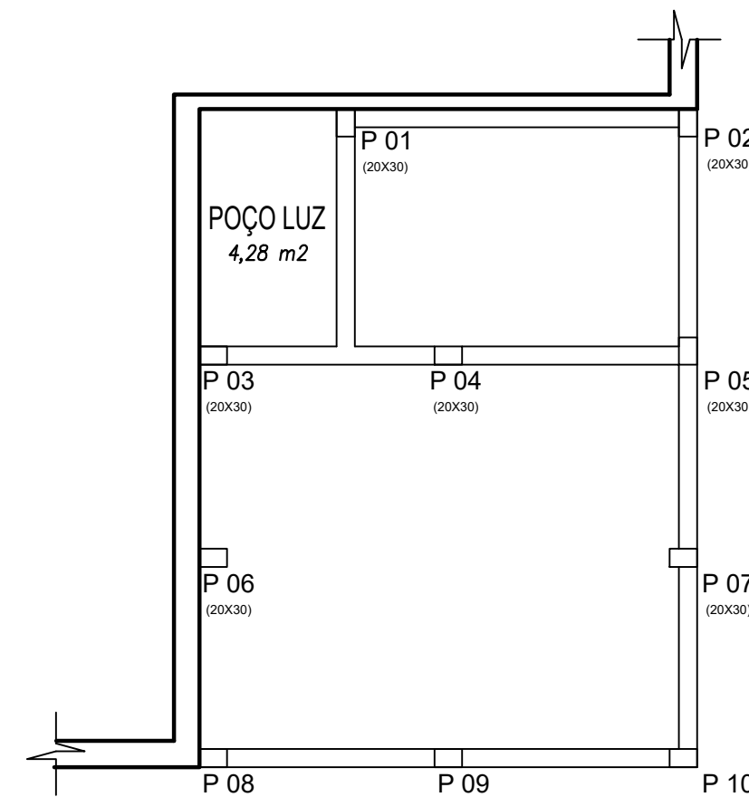
PLANTA BAIXA PILARES TÉRREO E PAV. SUPERIOR
