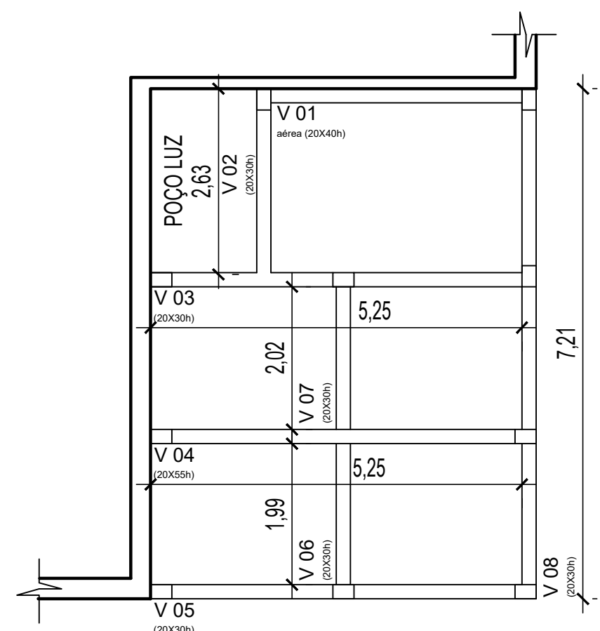
PLANTA BAIXA VIGA DE RESPALDO TÉRREO E PAV. SUPERIOR
