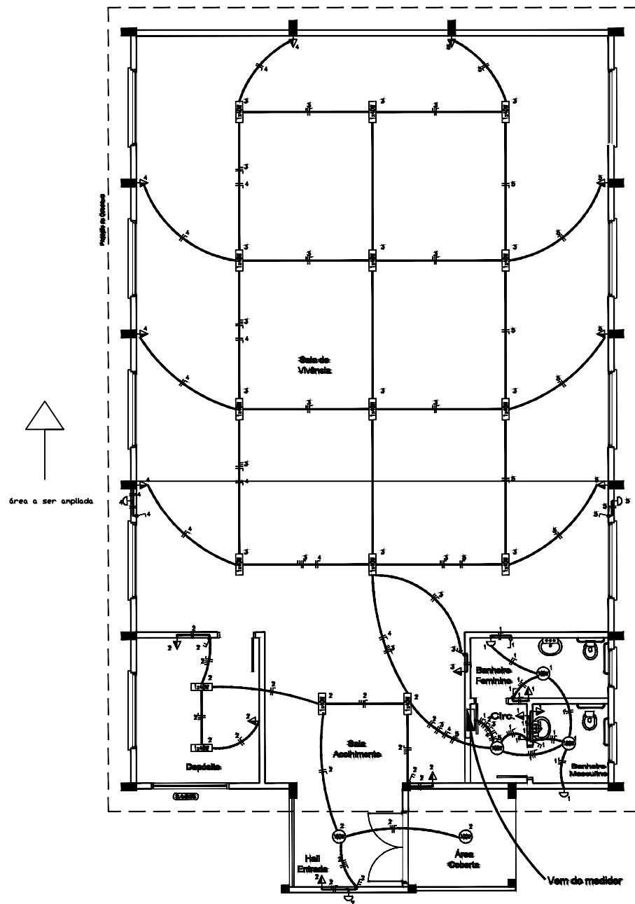
Planta Baixa Escala: 1/50
