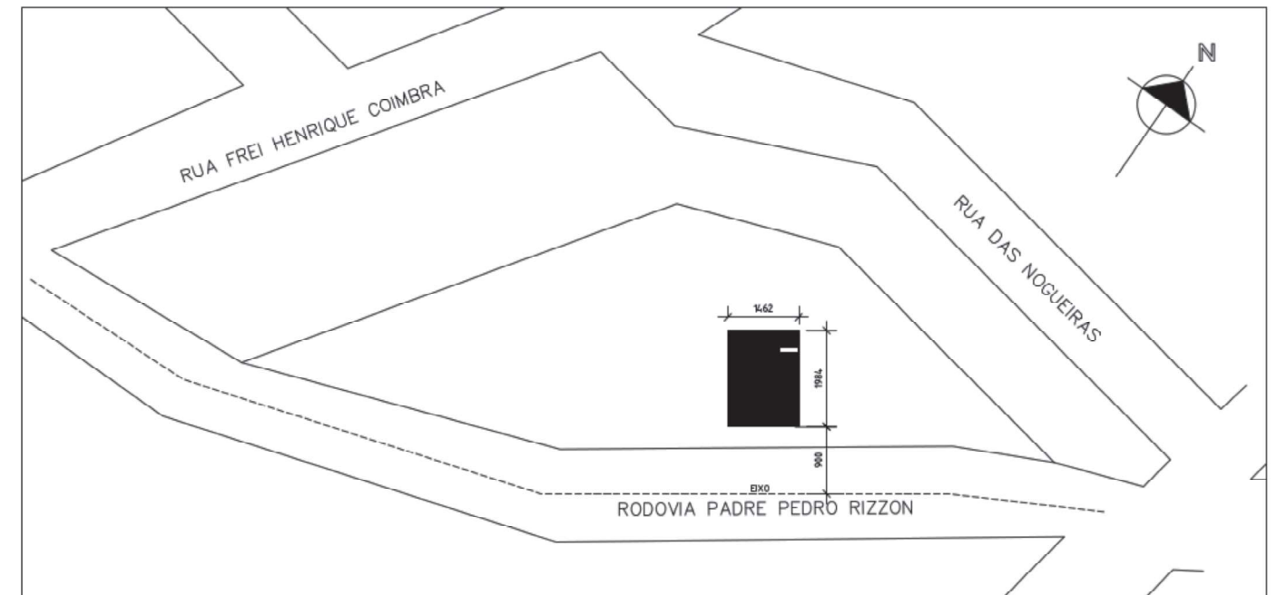
PLANTA DE SITUAÇÃO E LOCALIZAÇÃO Escala 1:1000
