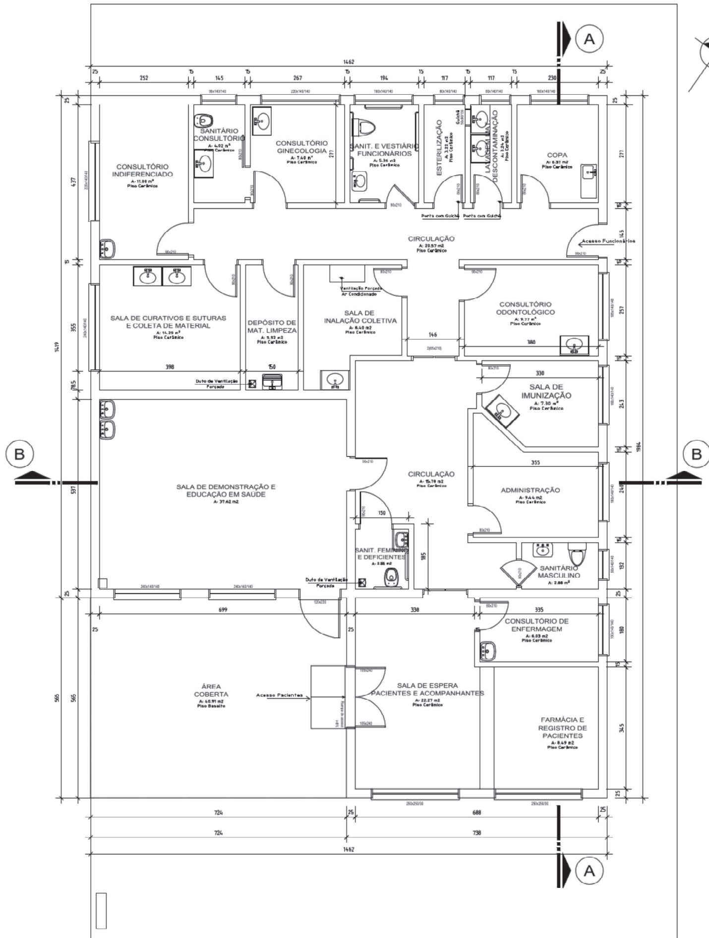
PLANTA BAIXA Escala 1:75 A: 290.06 m 2
