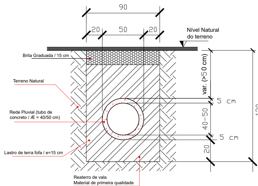
SEÇÃO TRANSVERSAL / Ø=40 cm
