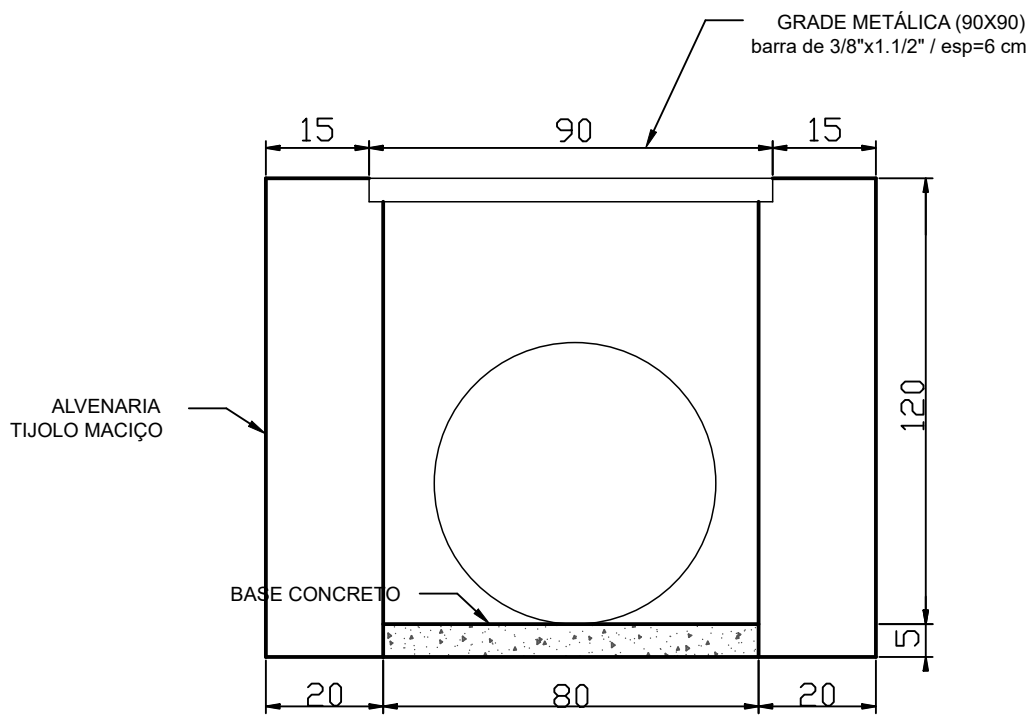
DETALHAMENTO DA BOCA DE LOBO (Ø= 40 cm)
