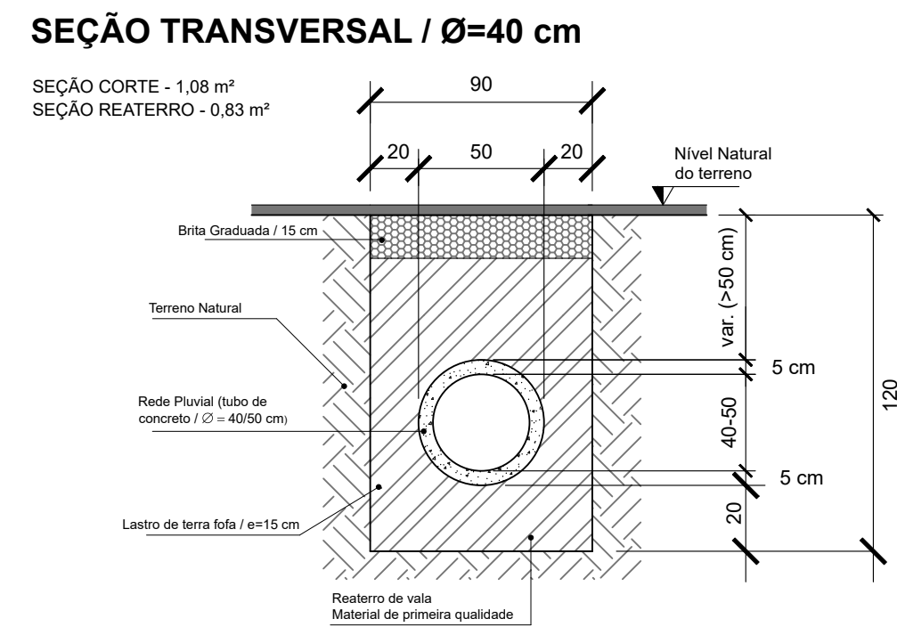
SEÇÃO TRANSVERSAL / Ø=40 cm
