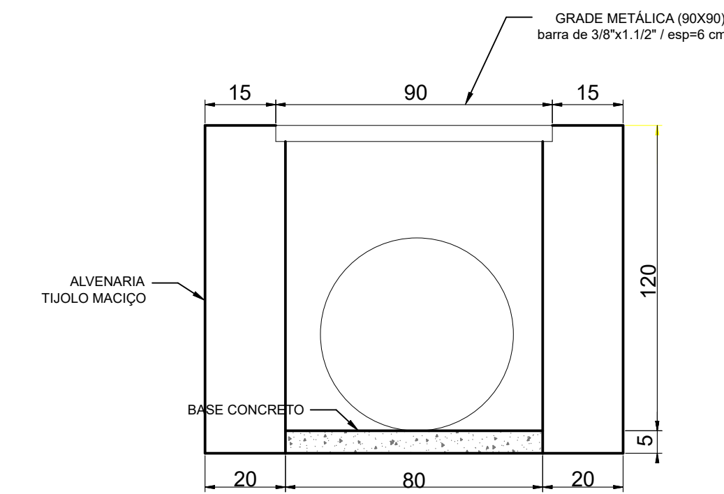
DETALHAMENTO DA BOCA DE LOBO (Ø= 40 a 60 cm)
