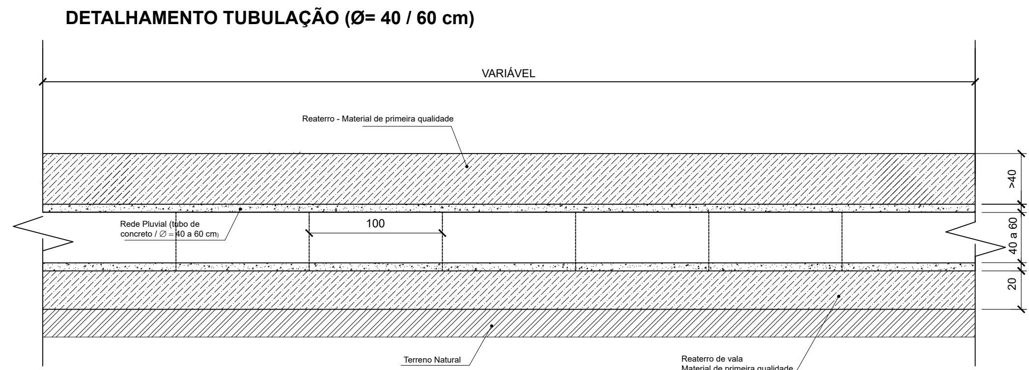
SEÇÃO LONGITUDINAL
