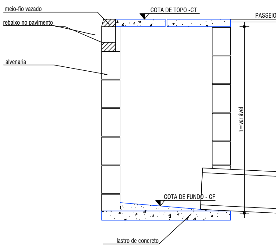
BOCA DE LOBO -CORTE AA ESC:1/25
