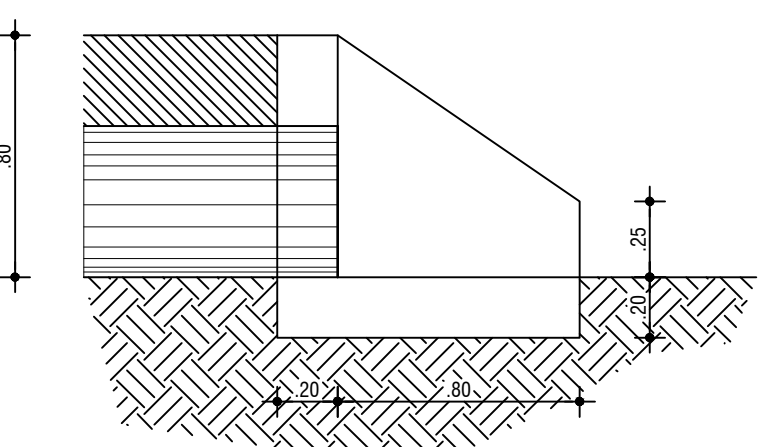
ALA Ø 400 -CORTE ESC:1/25
