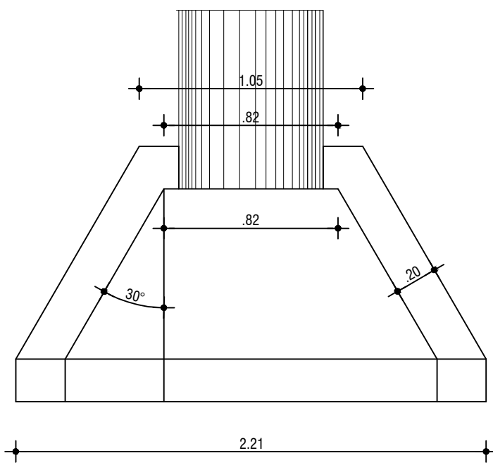
ALA Ø 600 - VISTA FRONTAL ESC:1/25
