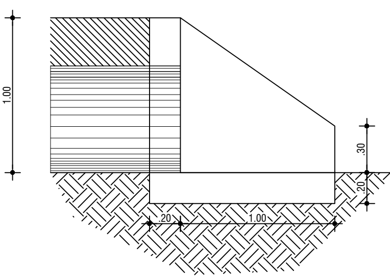
ALA Ø 600 -CORTE ESC:1/25
