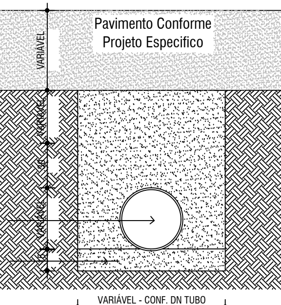
DETALHE - ESCAVAÇÃO E RECOBRIMENTO DE VALA ESC.: 1/25
