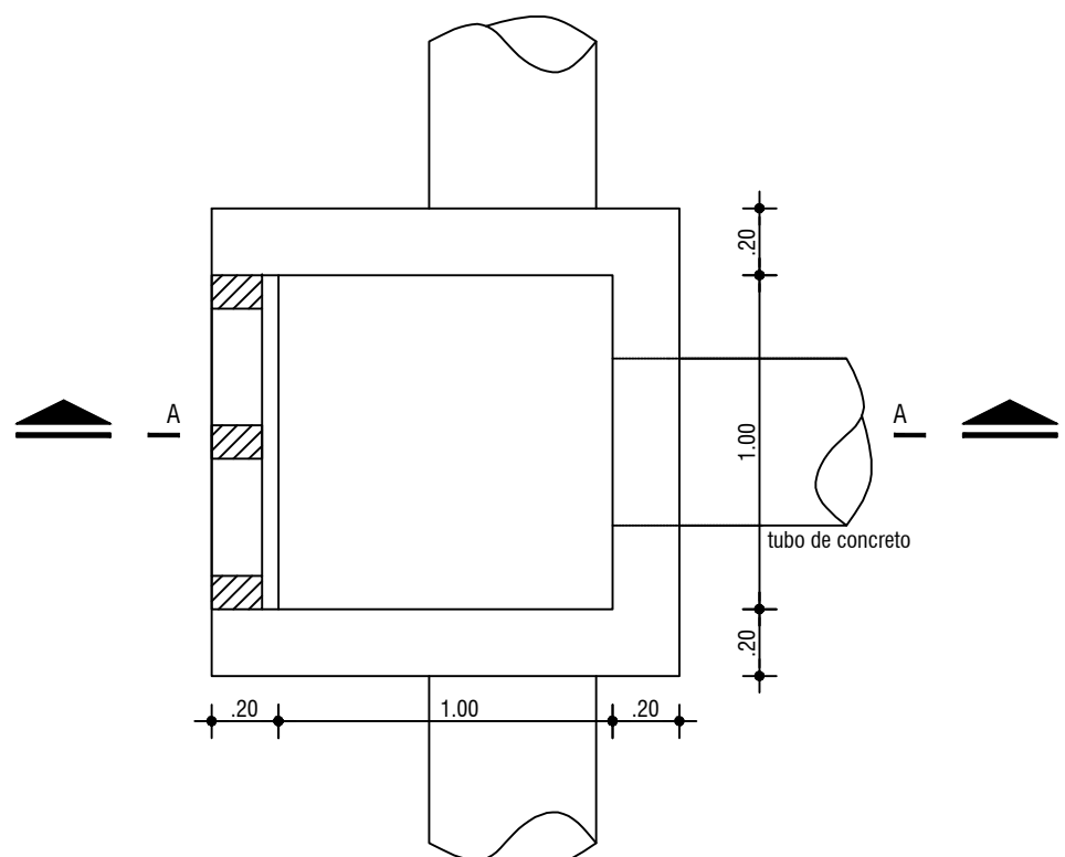
BOCA DE LOBO - PL. BAIXA ESC:1/25
