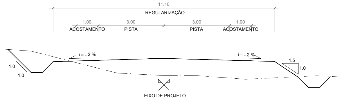
SEÇÃO TIPO DE TERRAPLENAGEM Sem escala
