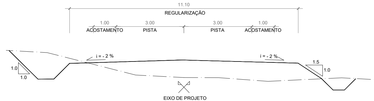
SEÇÃO TIPO DE TERRAPLENAGEM Sem escala
