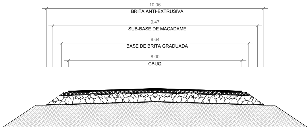
SEÇÃO TIPO DE PAVIMENTAÇÃO Sem escala
