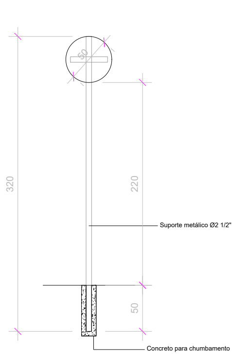
PLACA DE REGULAMENTAÇÃO Sem escala
