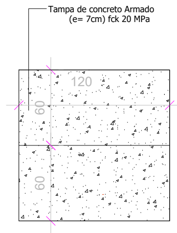
PLANTA BAIXA - TAMPA Sem escala
