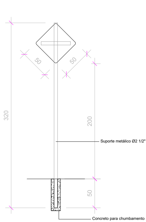
PLACA DE ADVERTÊNCIA Sem escala
