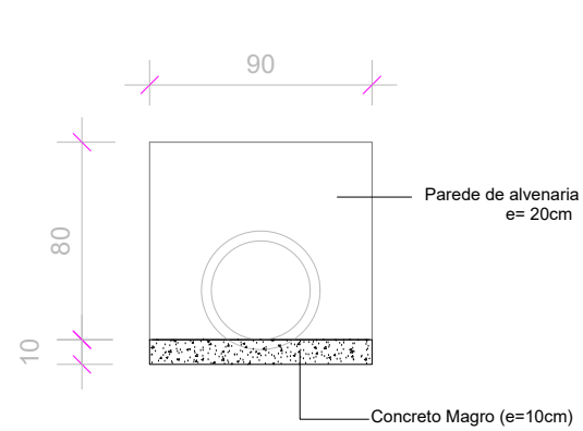
VISTA FRONTAL Sem escala TESTADA PARA BUEIRO Ø400mm Sem escala
