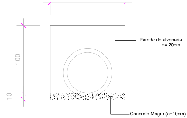
VISTA FRONTAL Sem escala TESTADA PARA BUEIRO Ø600mm Sem escala
