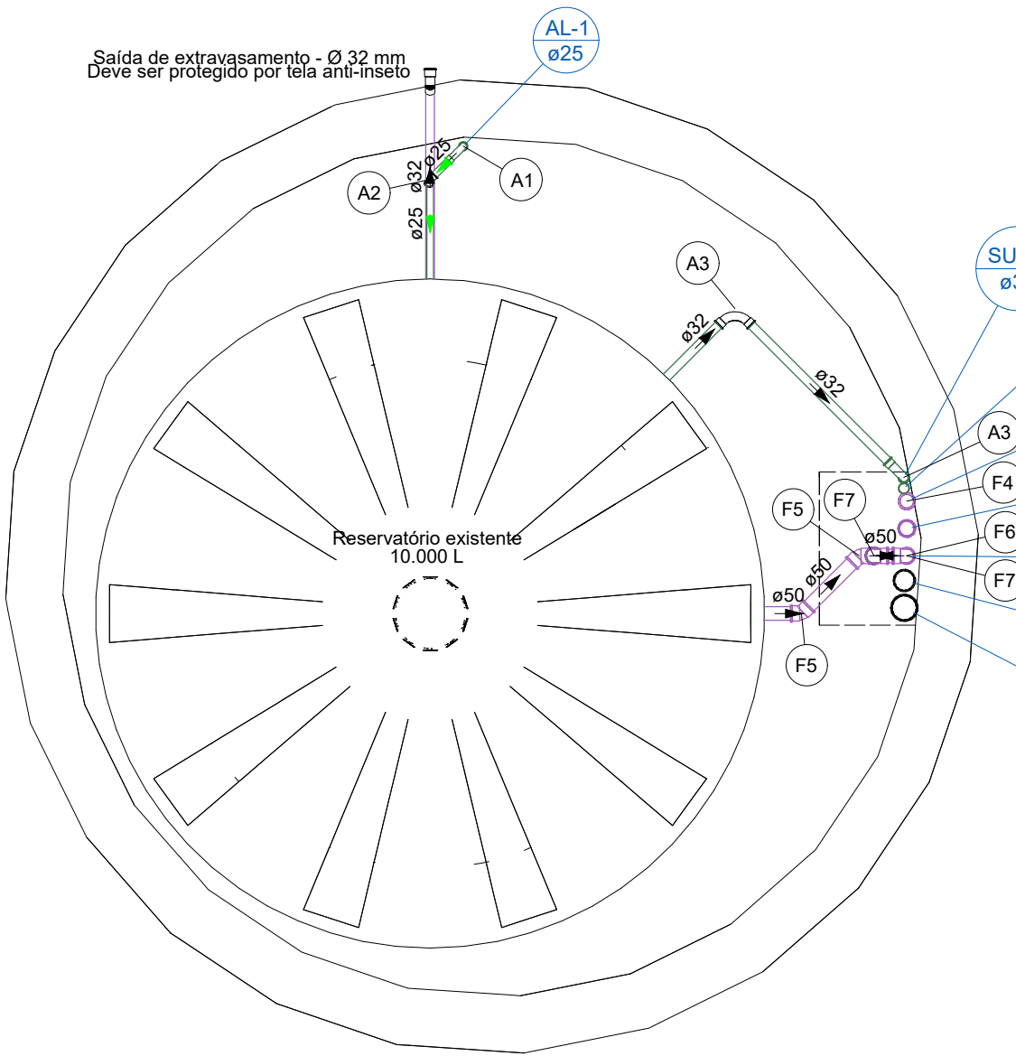
PLANTA BAIXA - 1º PAVIMENTO - RESERVATÓRIO 1 - CISTERNA
