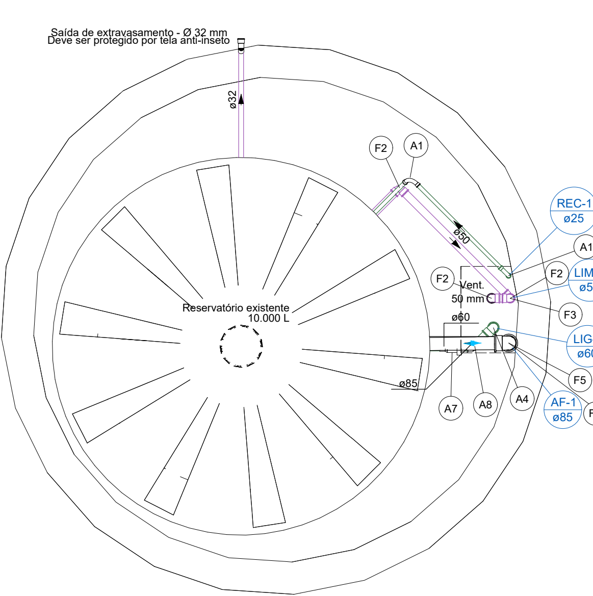
PLANTA BAIXA - 3º PAVIMENTO - RESERVATÓRIO 3 - CONSUMO
