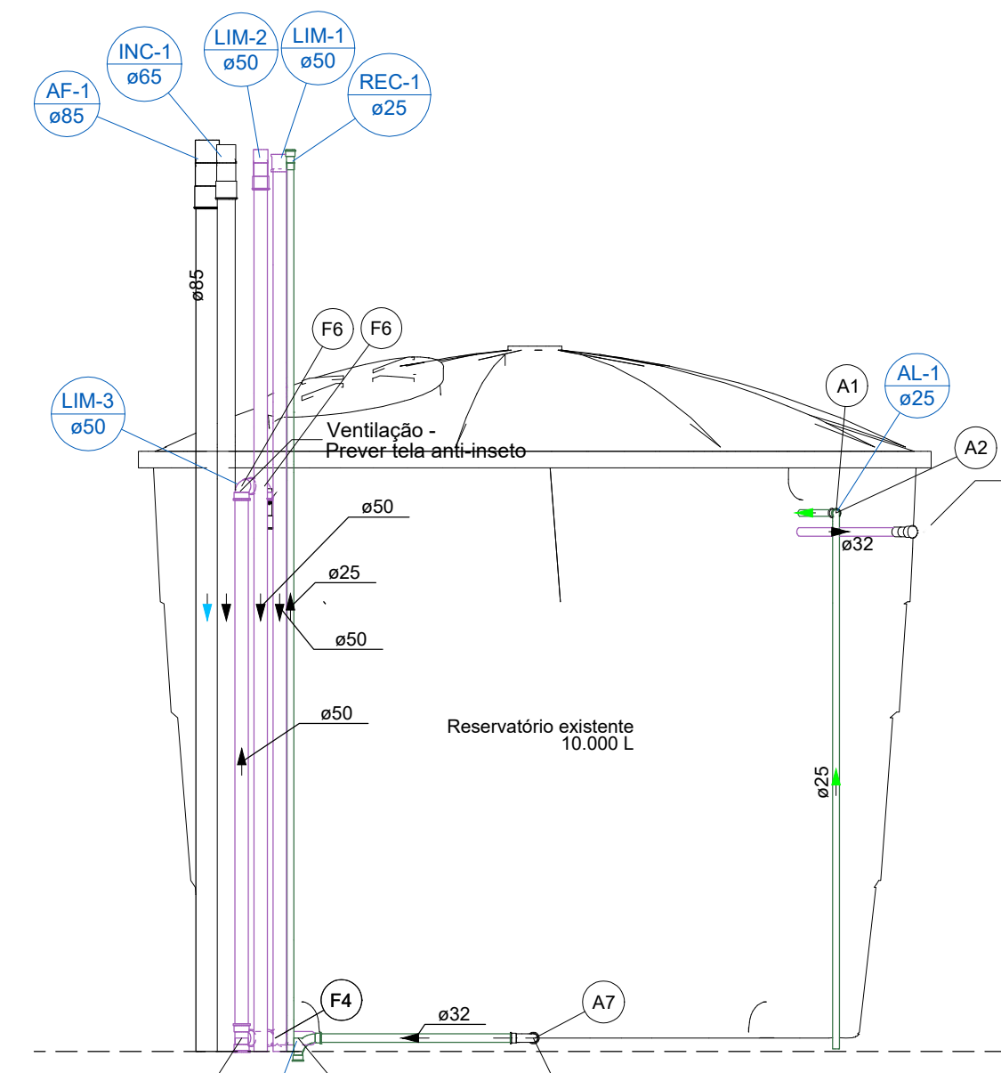
CORTE - 1º PAVIMENTO - RESERVATÓRIO 1 - CISTERNA
