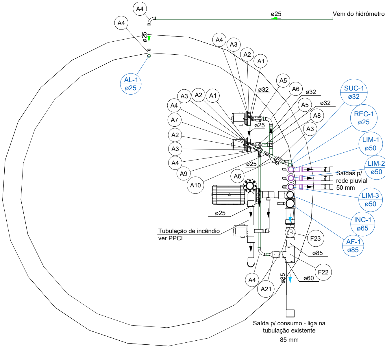
PLANTA BAIXA - TÉRREO - CASA DE MÁQUINAS
