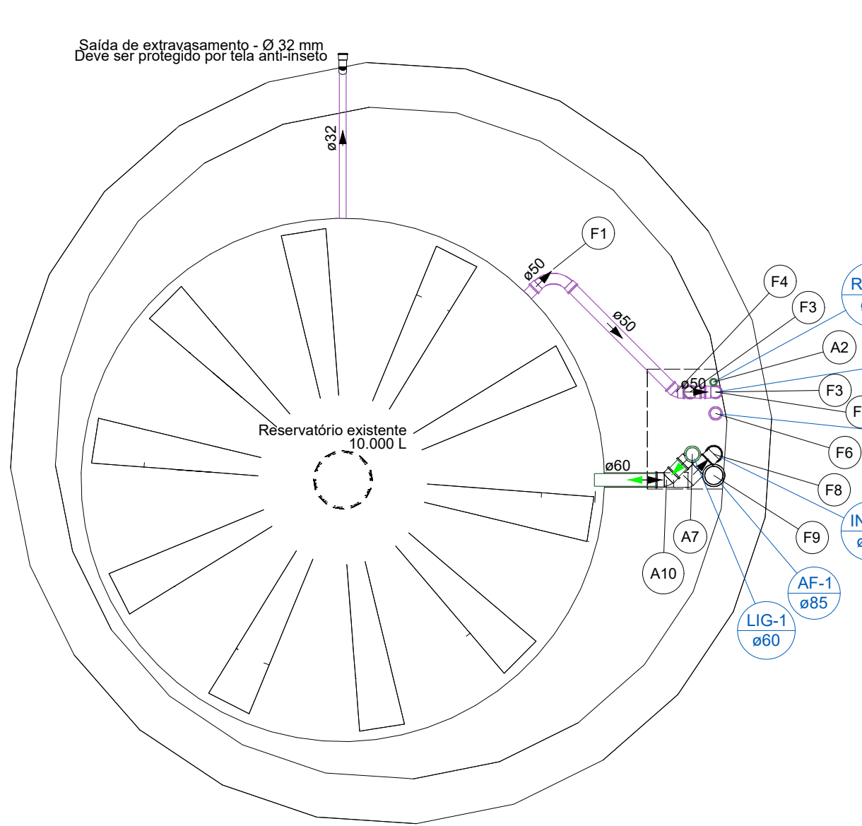
PLANTA BAIXA - 2º PAVIMENTO - RESERVATÓRIO 2 - RTI
