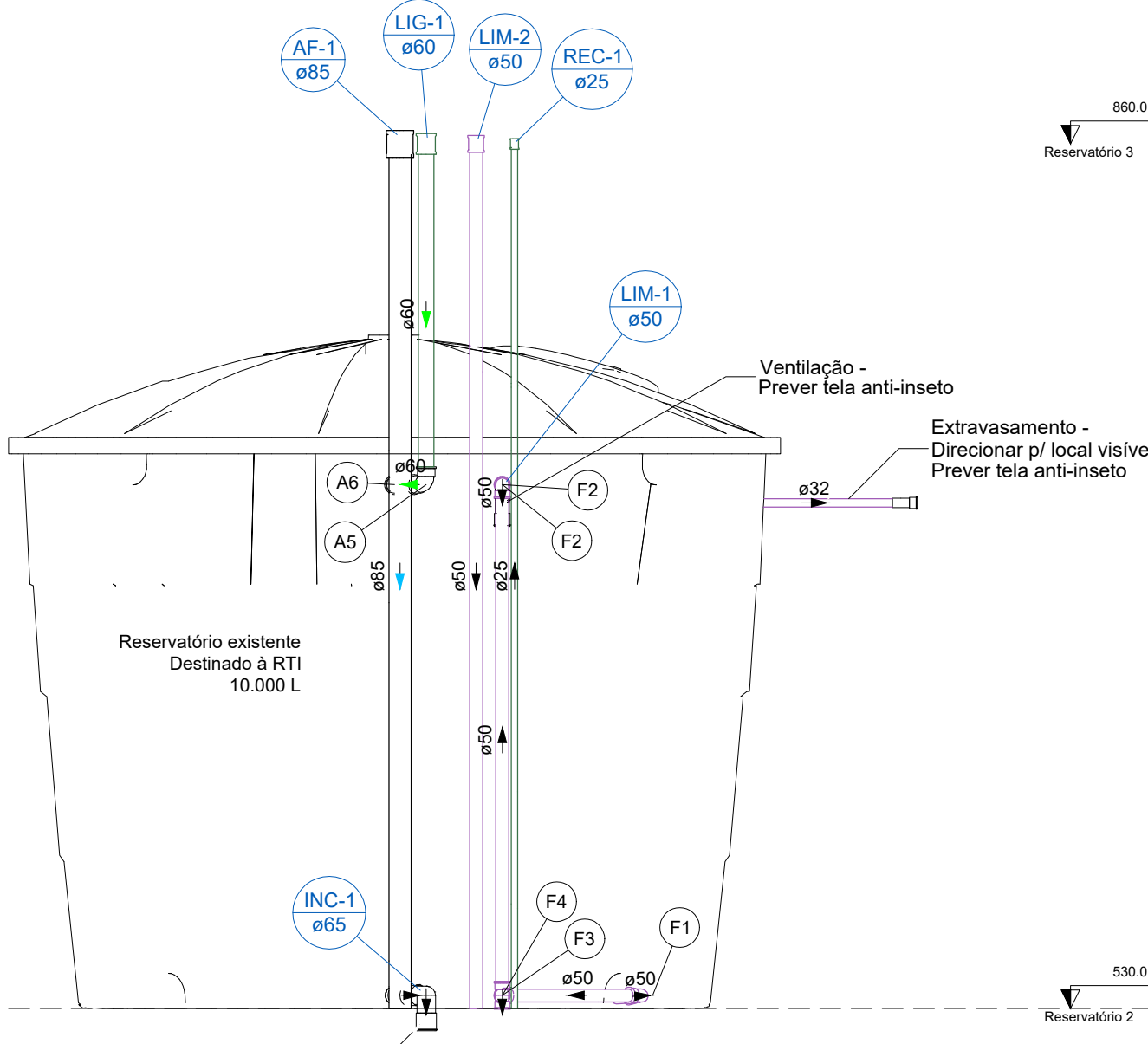
CORTE - 2º PAVIMENTO - RESERVATÓRIO 2 - RTI
