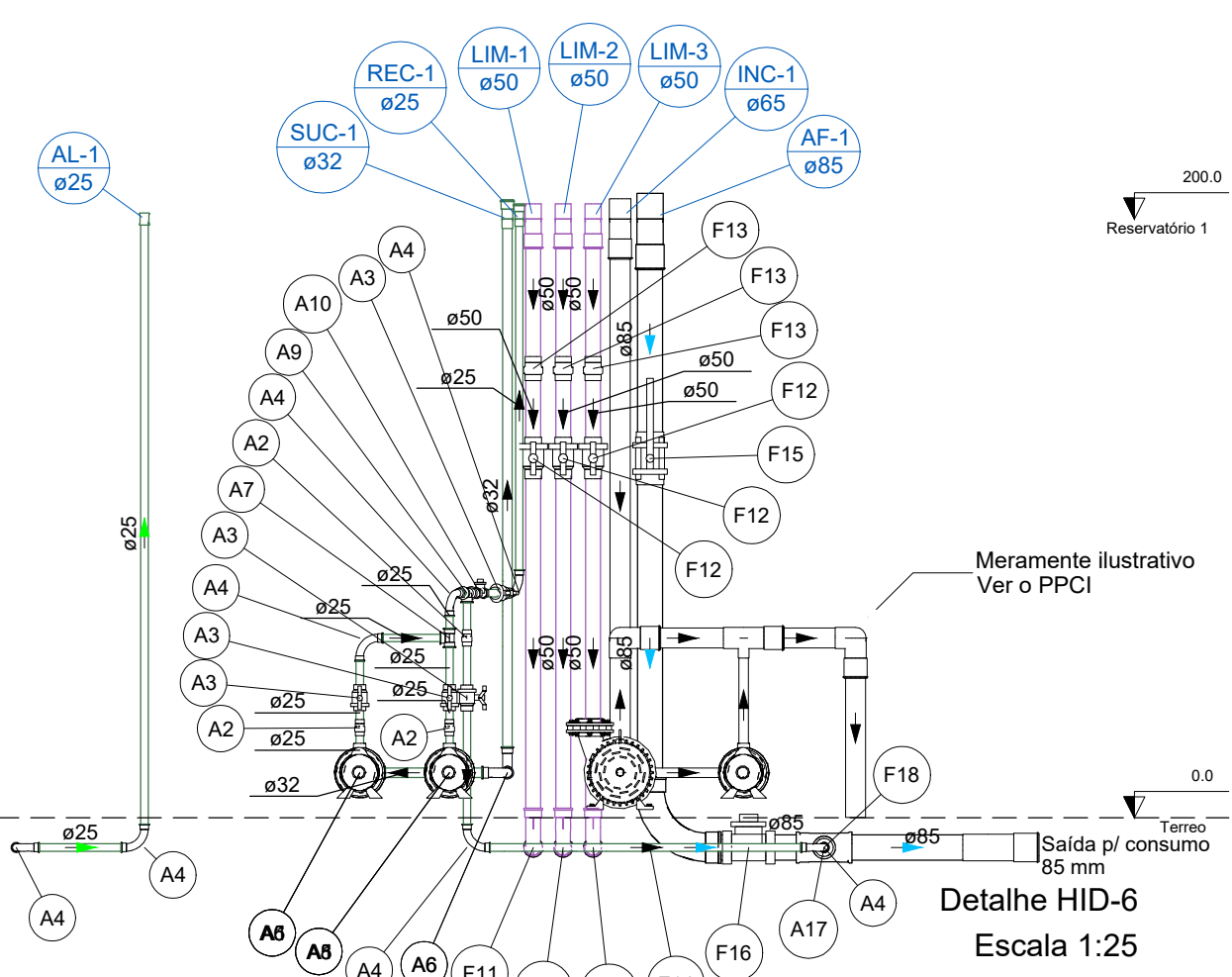
CORTE - TÉRREO - CASA DE MÁQUINAS
