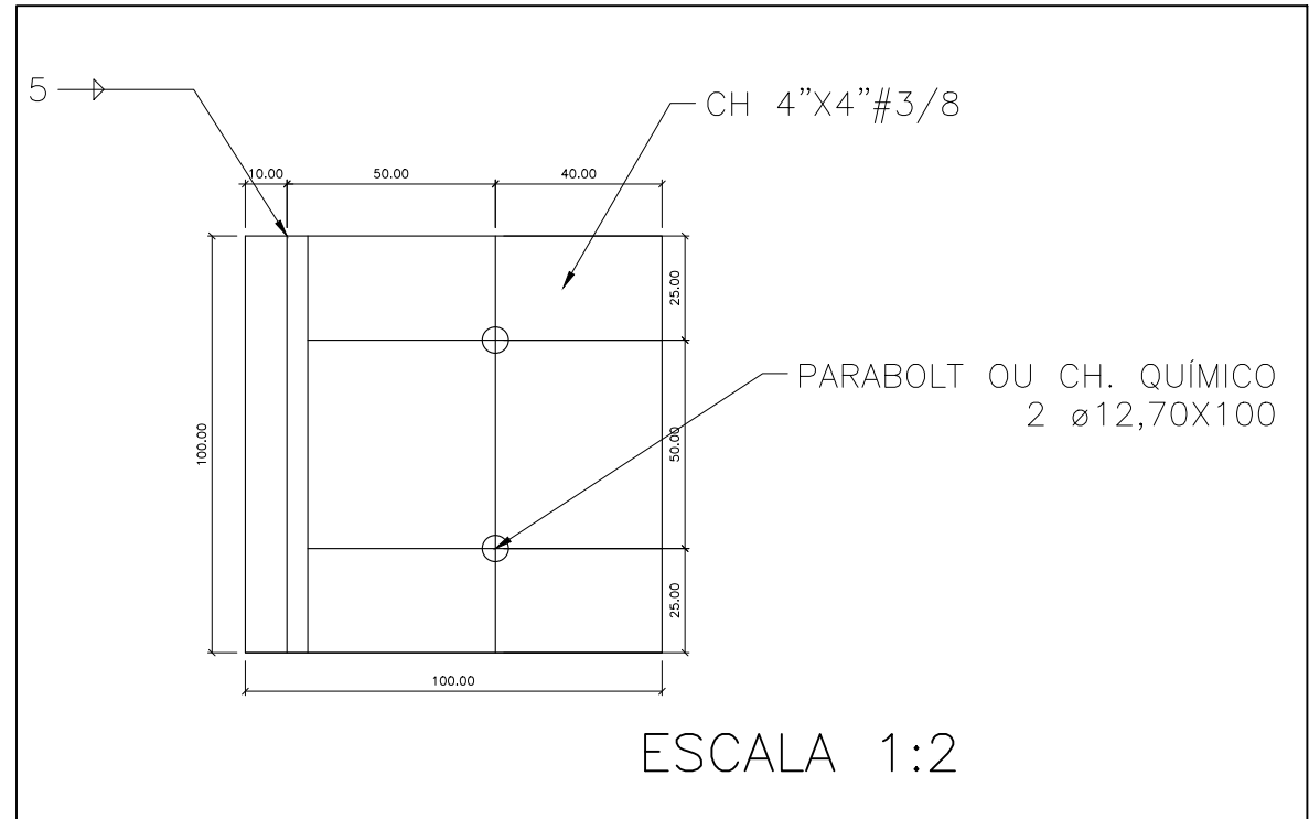
DETALHE A – PLACA DE BASE – APOIO GUARDA CORPO NA ALVENARIA
