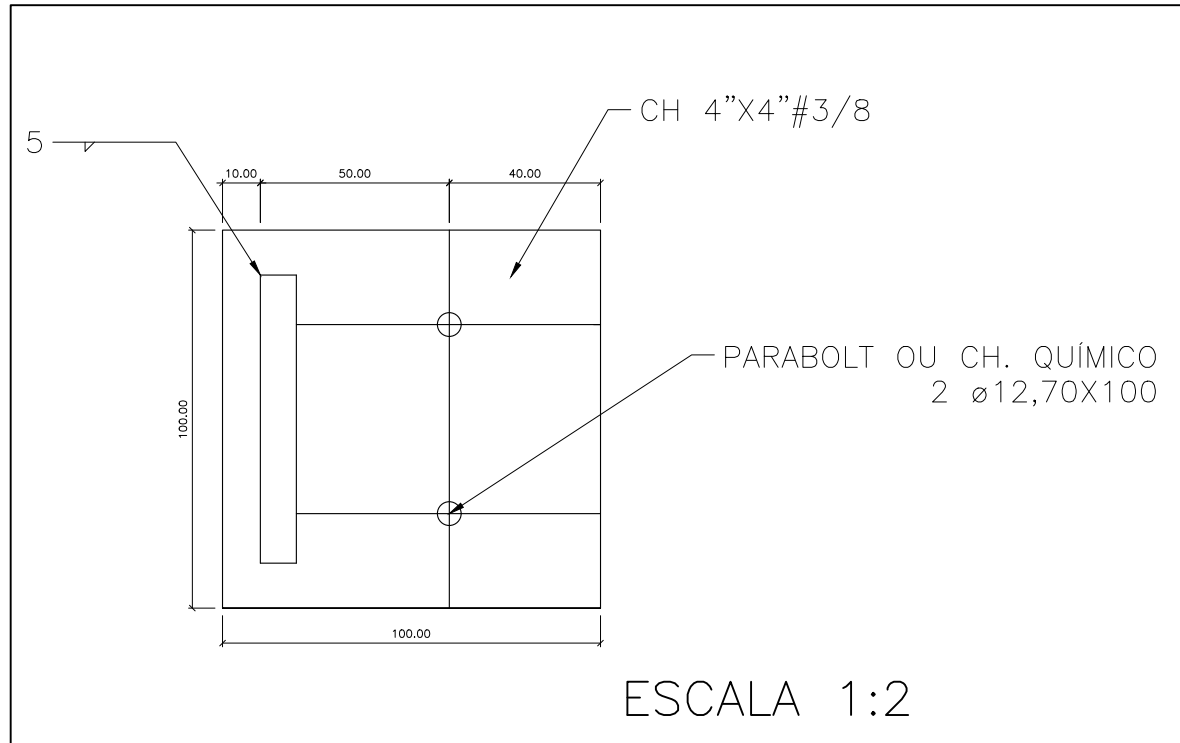
DETALHE C – PLACA DE BASE DO PASSA-MÃO
