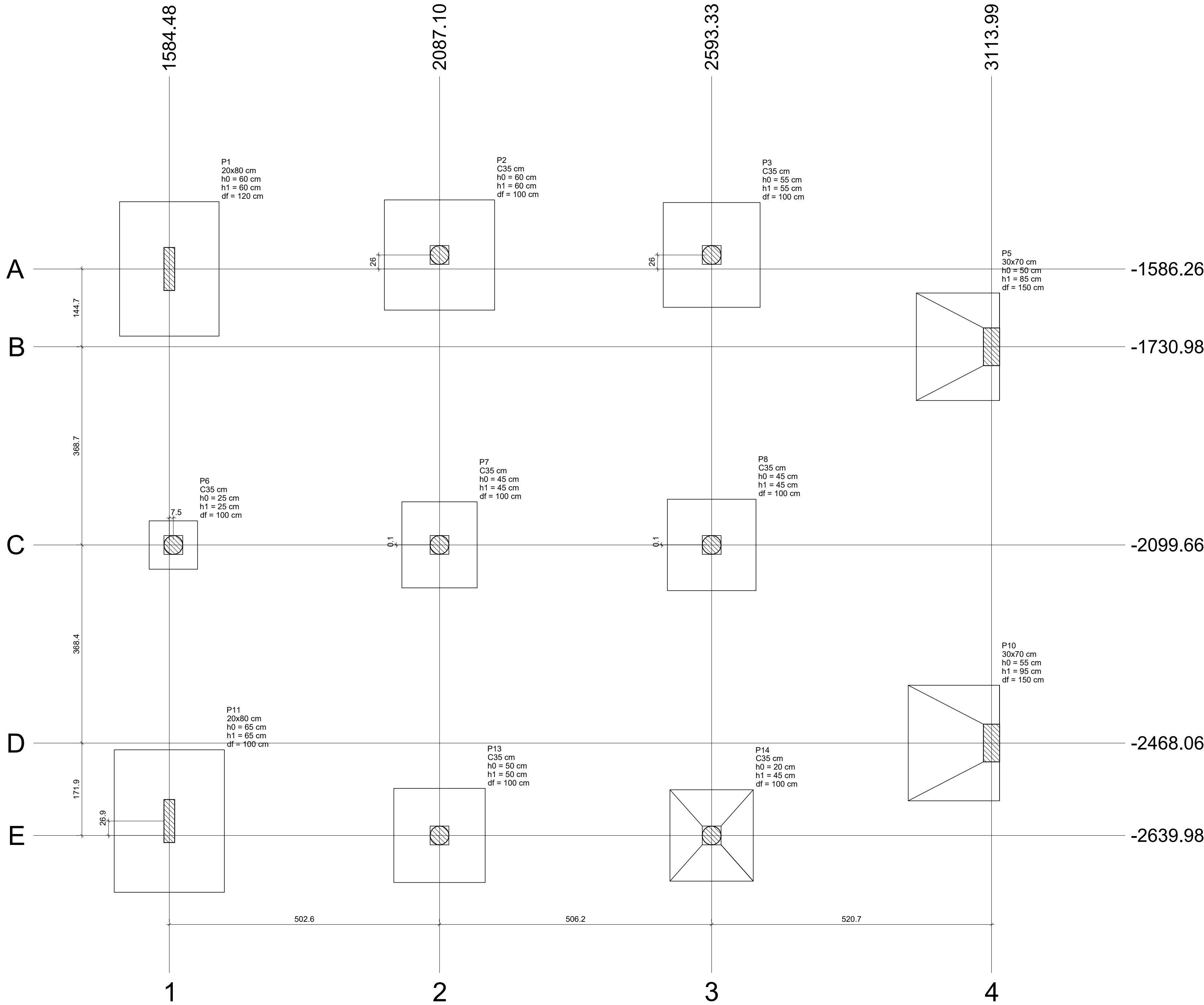
Planta de locação escala 1:50
