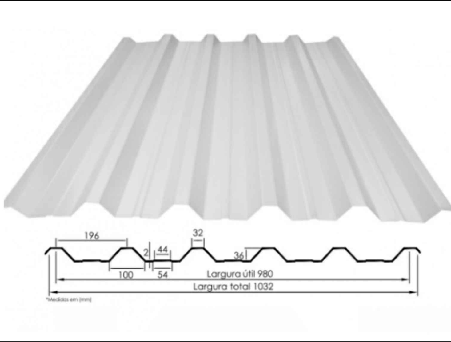
DETALHE TELHA TP40 TERMOACÚSTICA COM PREENCHIMENTO EM PU
