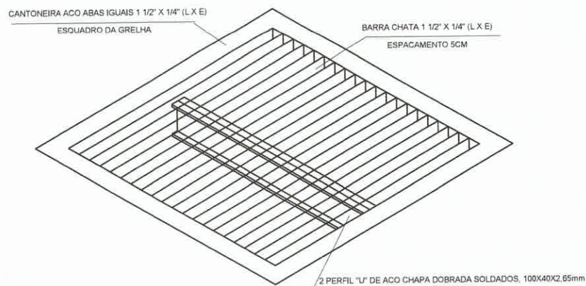
Tampa Metálica - Barra chata Esc: Sem escala
