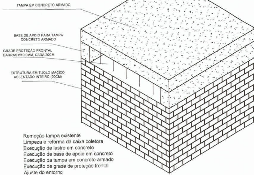
Caixa coletora com tampa em concreto Esc: Sem escala
