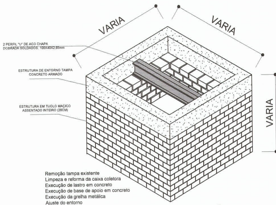
Caixa coletora para grelha Esc: Sem escala
