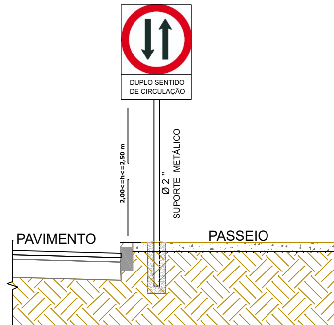
DETALHE INST. PLACAS DE SINALIZAÇÃO SIMPLES SEM ESCALA
