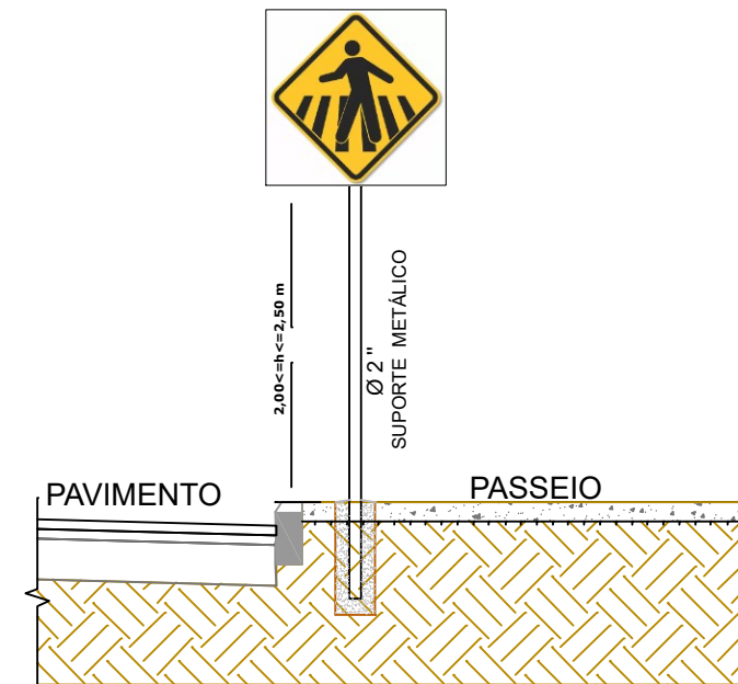
DETALHE INST. PLACAS DE SINALIZAÇÃO SIMPLES SEM ESCALA
