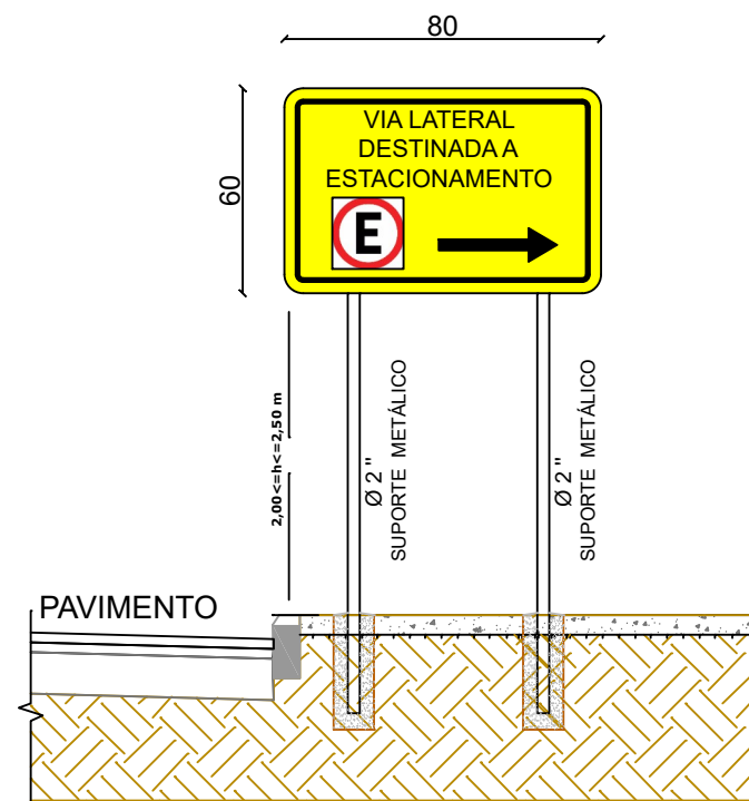
DETALHE INST. PLACAS DE SINALIZAÇÃO SEM ESCALA
