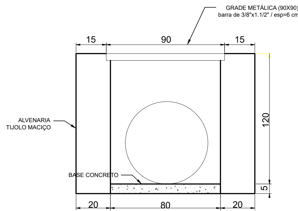
DETALHAMENTO DA BOCA DE LOBO (Ø= 40 a 60 cm)
