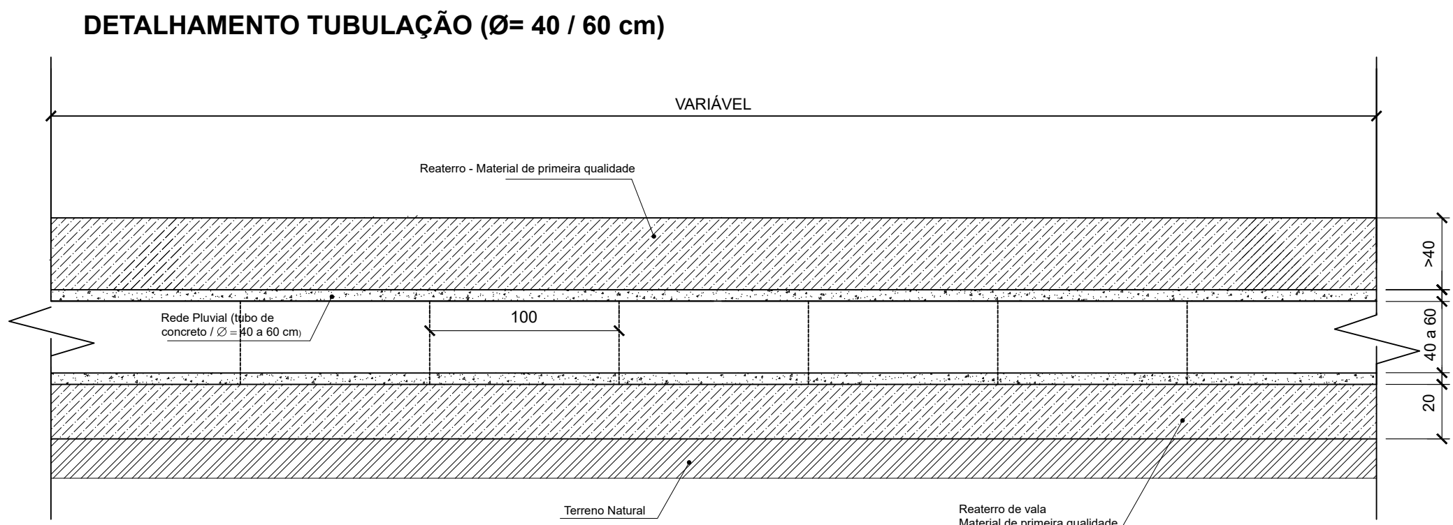
SEÇÃO LONGITUDINAL
