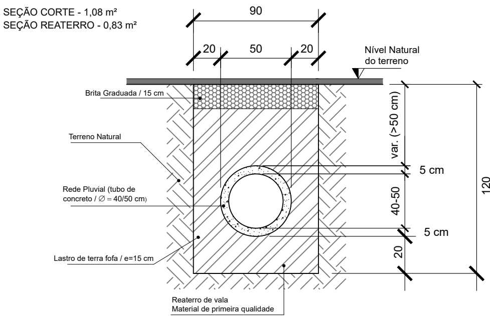
SEÇÃO TRANSVERSAL / Ø=40 cm
