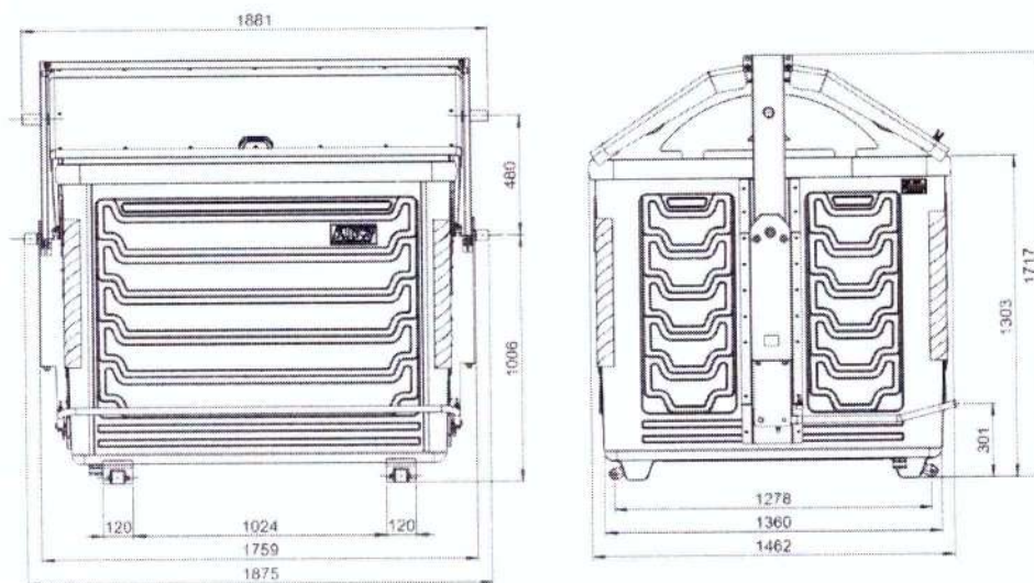
Dimensões - Contentor Metálico 3,20m³ - BUSA
