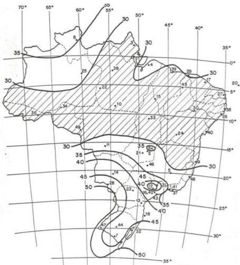
Figura 8: Isopletas de velocidades básicas do vento (m/s)
