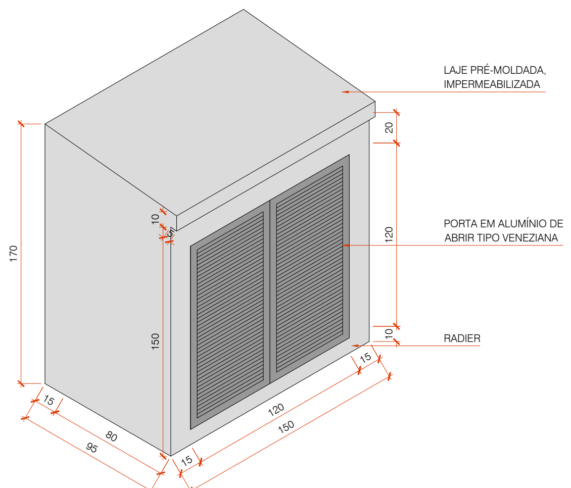
4 DETALHE ABRIGO DO COMPRESSOR Esc.: 1/25
