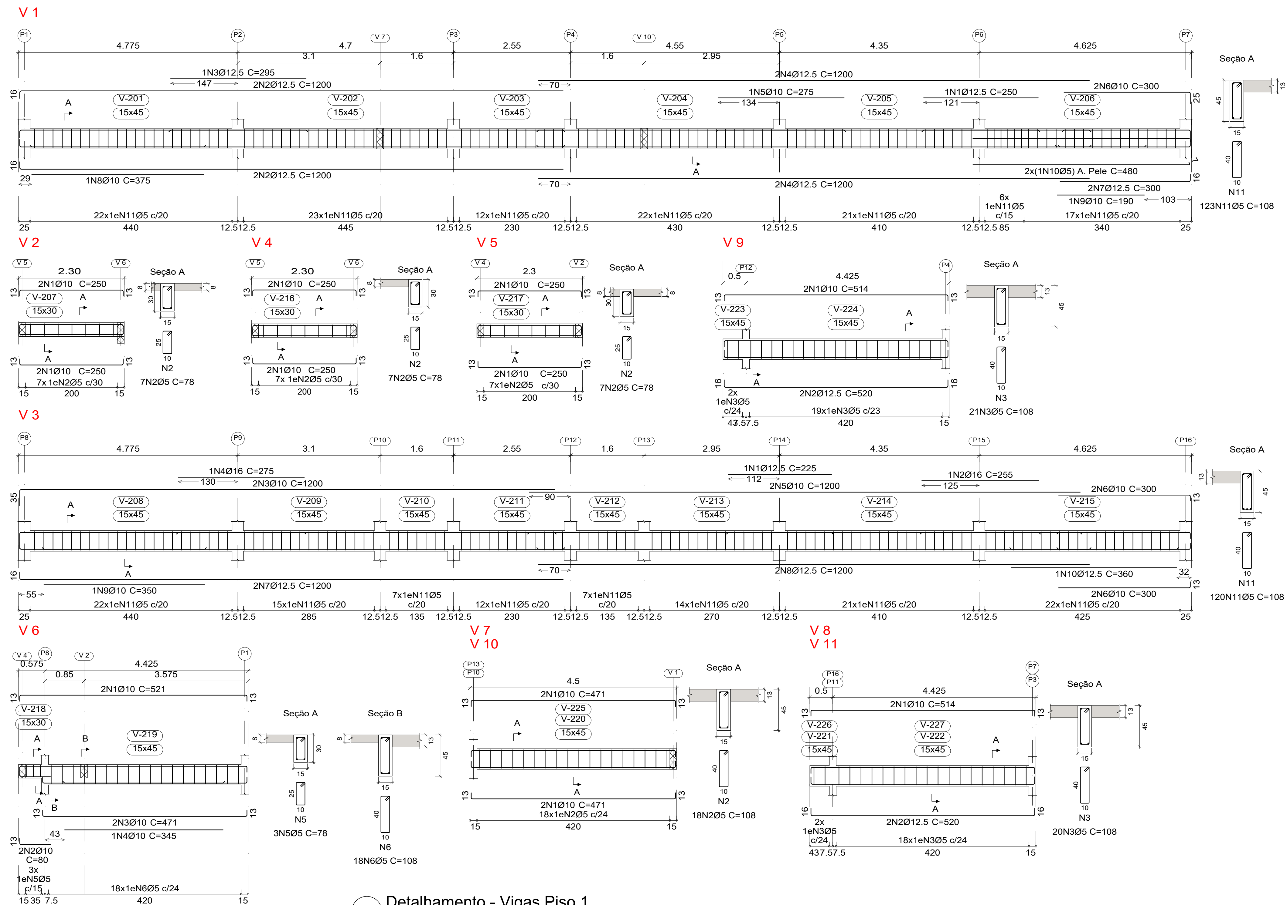
11.2 Detalhamento - Vigas Piso 1 Escala: 1/50
