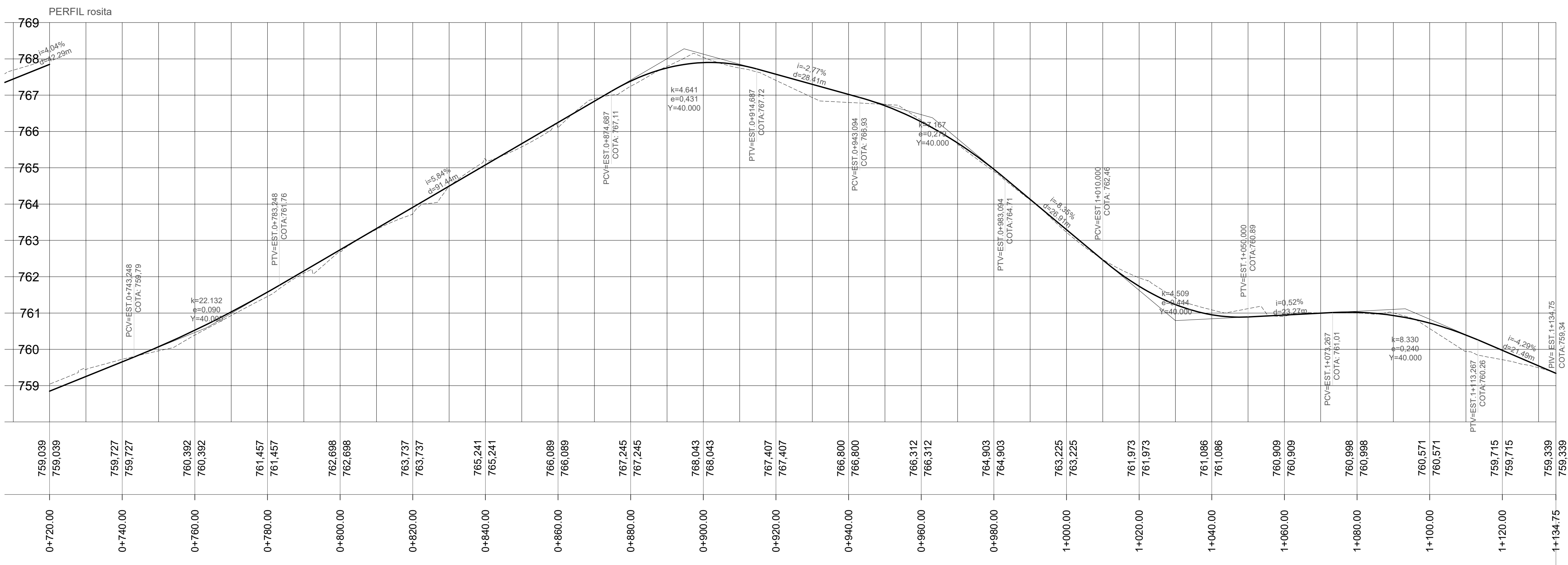
03 Perfil Longitudinal Escala: 1/700
