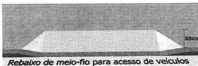
Figura 2 – rebaixo de meio-fio
