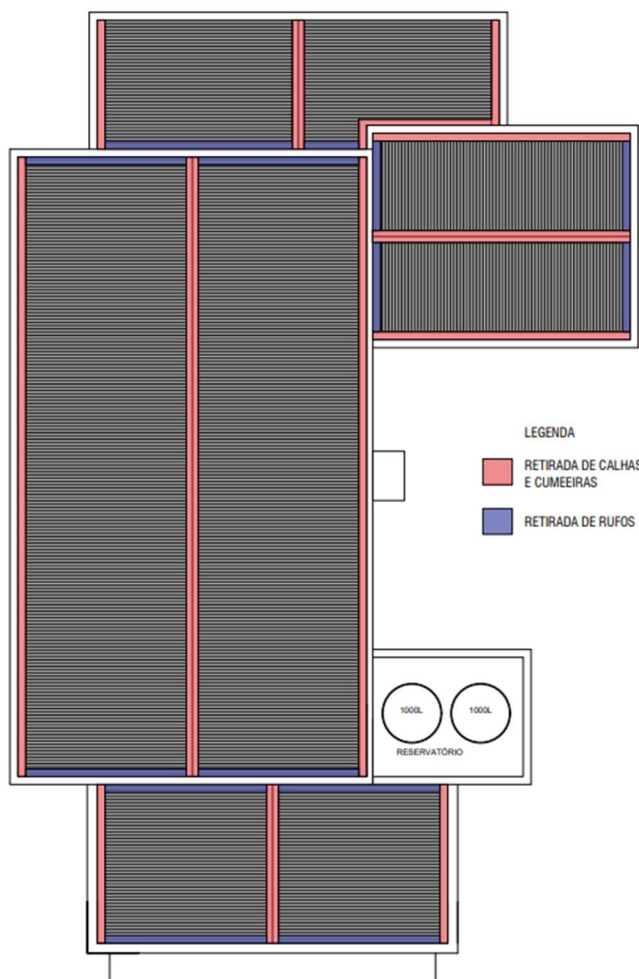
Planta esquemática – sem escala O serviço de remoção de capa metálica é medido por m^2 .
