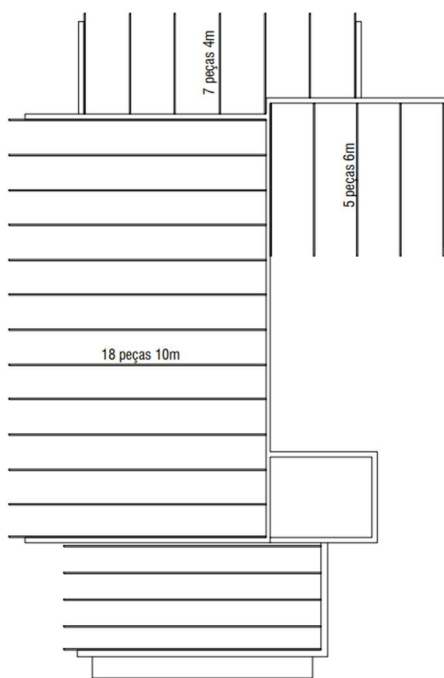
Planta esquemática – sem escala.
