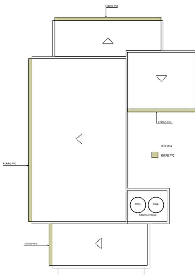
Planta esquemática – sem escala O serviço será medido em m² de forro instalado.
