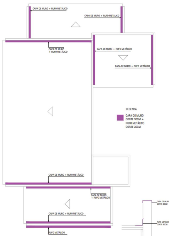
Planta esquemática – sem escala O serviço será medido em m linear de rufo instalado.
