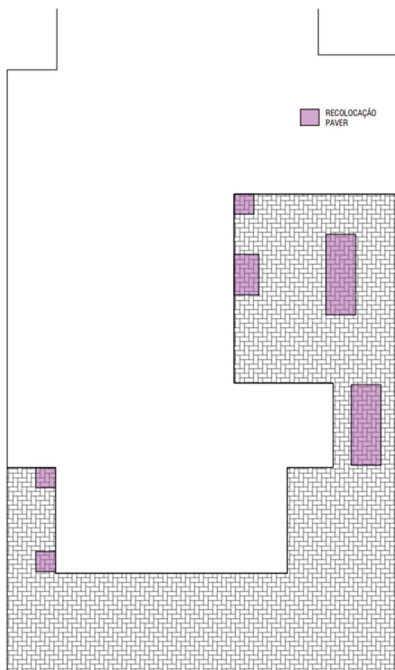
Planta esquemática – sem escala O serviço será medido por m 2 de paver reinstalado.
