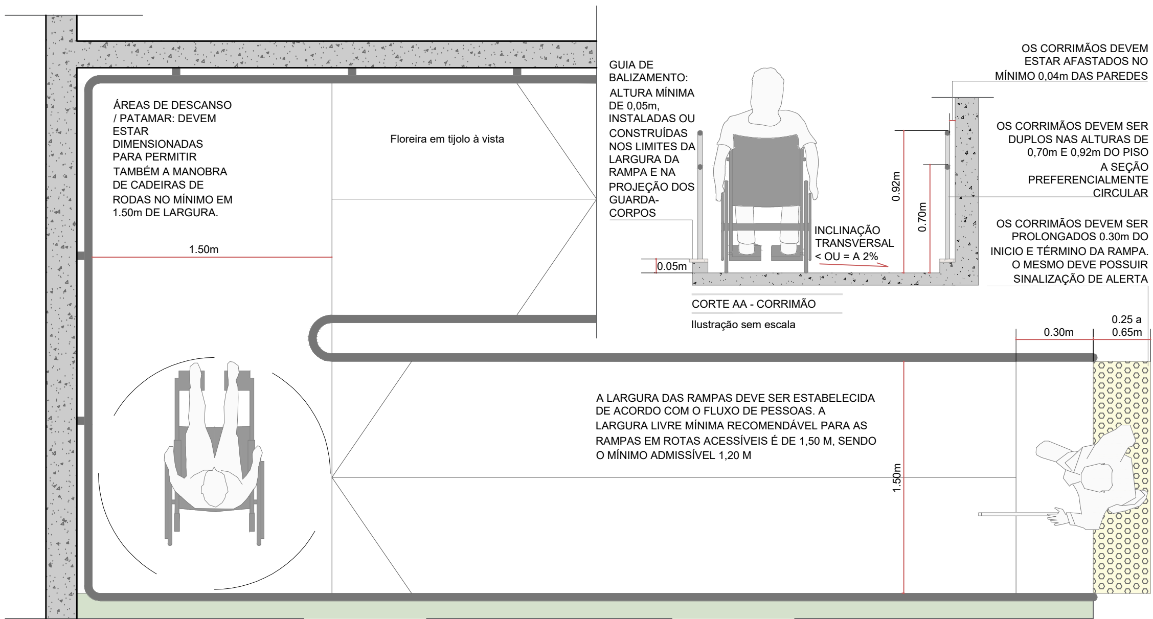
RAMPA ACESSÍVEL - ORIENTAÇÕES GERAIS CONFORME NBR 9050
