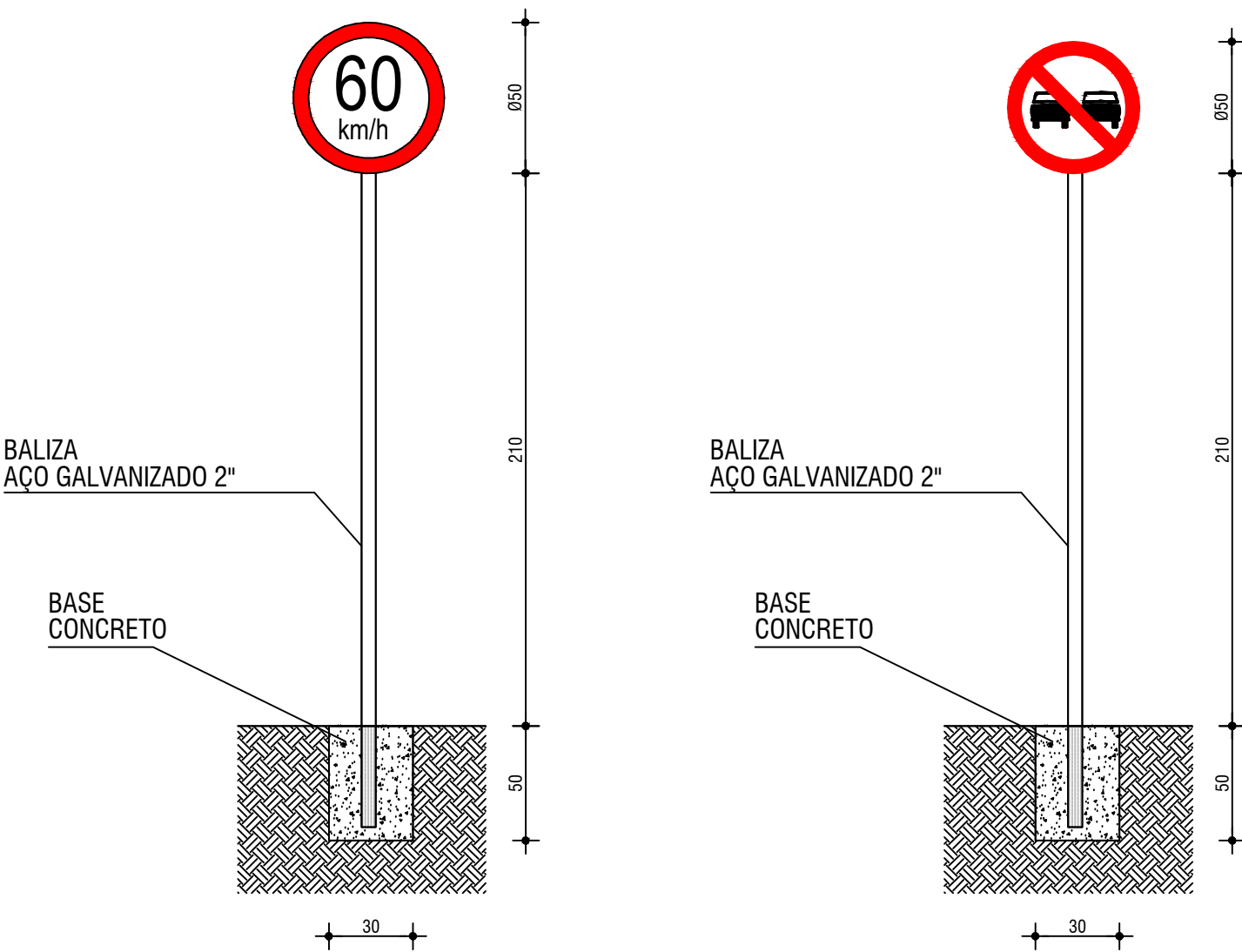
DETALHE SINALIZAÇÃO ESC:1/25
