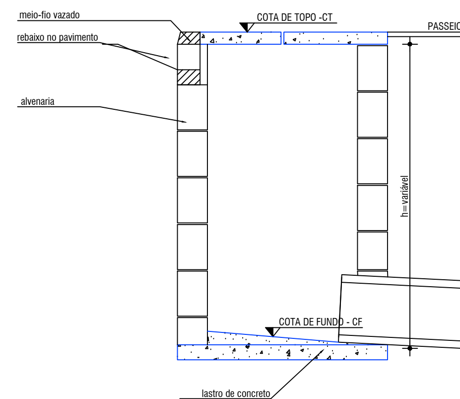
BOCA DE LOBO -CORTE AA ESC:1/25
