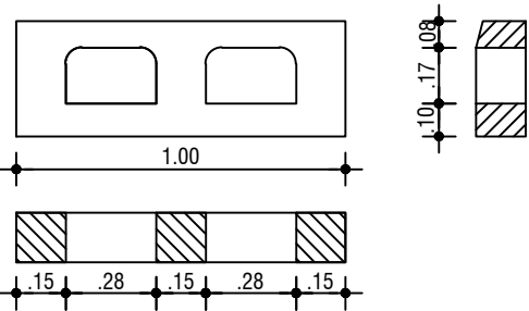
DETALHE BOCA-DE-LOBO - MEIO-FIO ESC:1/25
