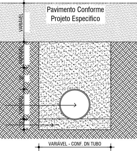
TUBO DE ESGOTO PLUVIAL DN CONFORME PROJETO ÁREA MÉDIA
