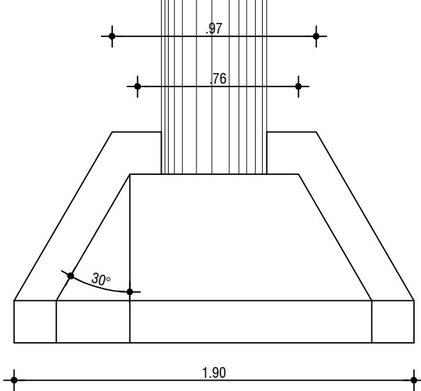
ALA Ø 400 - VISTA FRONTAL ESC:1/25
