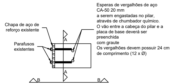
PLANTA BAIXA - CABEÇA DO PILAR Sem Escala
