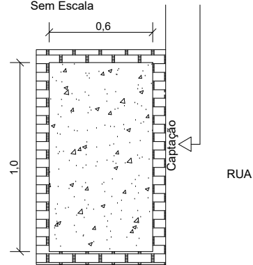
VISTA SUPERIOR Sem Escala
