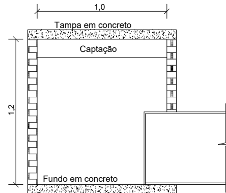
VISTA EM CORTE Sem Escala
