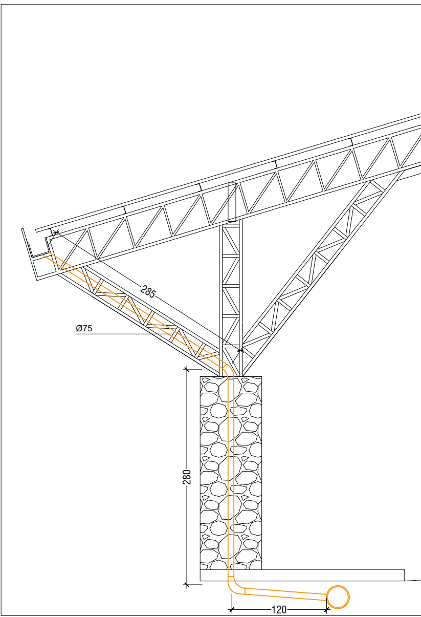
Esquema tubo de queda pluvial Esc. 1/50
