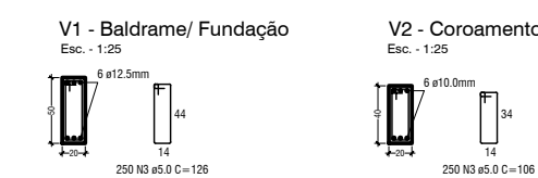
Detalhamento Vigas Coroamento
