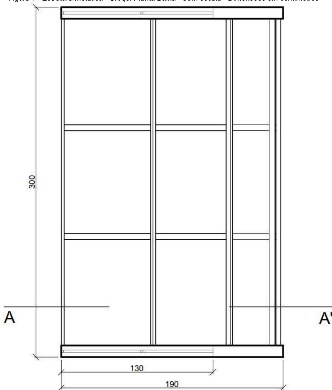
Figura 1 - Estrutura Metálica - Croqui Planta Baixa - Sem escala - Dimensões em centímetros
