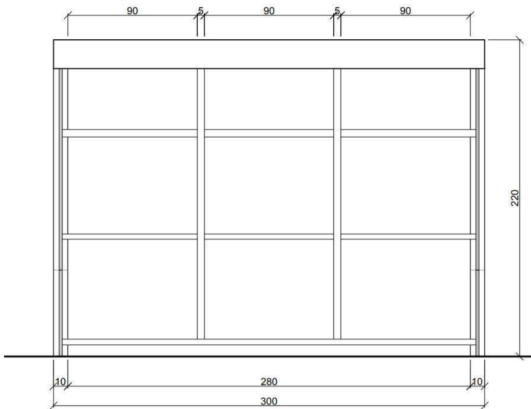
Figura 3 - Estrutura Metálica - Croqui Vista Frontal - Sem escala - Dimensões em centímetros
